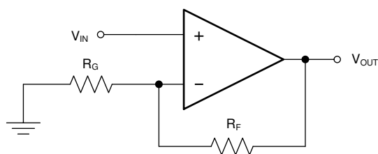
图 8-3. OPA392 布局原理图
