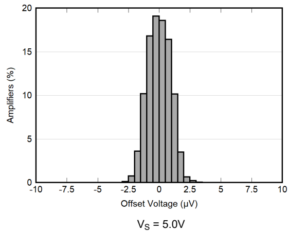
图 6-1. 失调电压分布图
