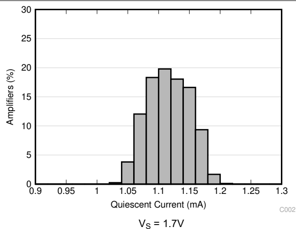
图 6-8. 静态电流分布
