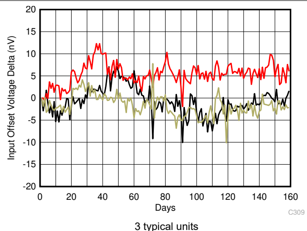
图 6-6. Offset Voltage Long Term Drift
