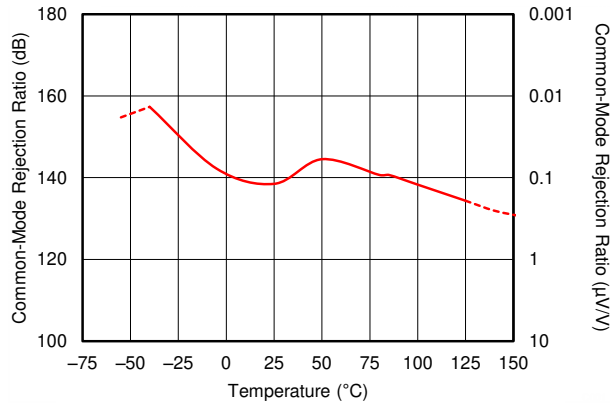
图 6-13. CMRR vs Temperature
