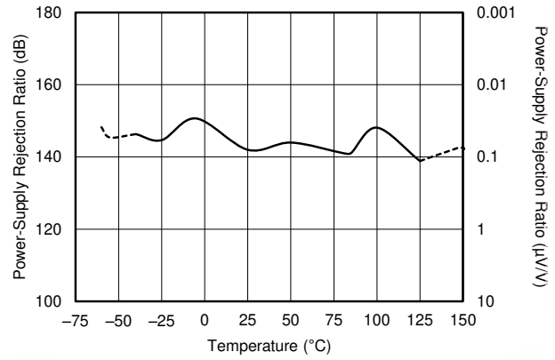
图 6-14. PSRR vs Temperature
