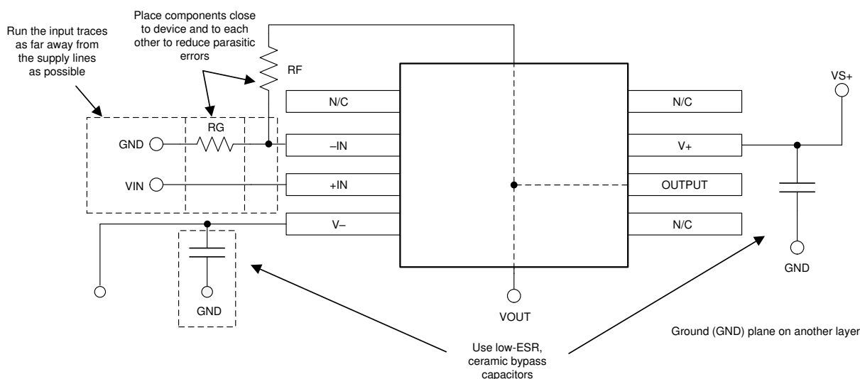
图 10-2. Layout Example
