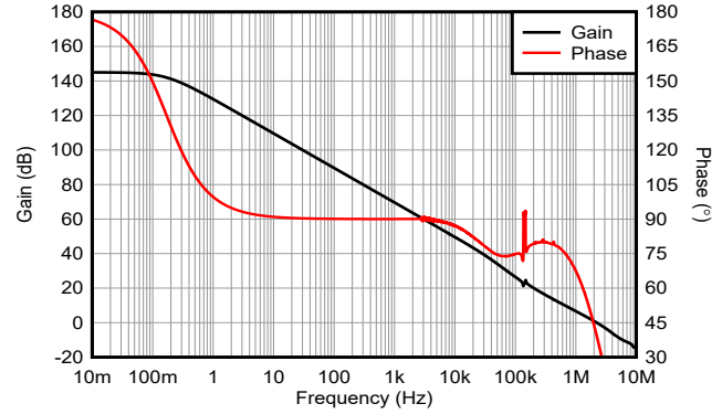
图 5-8. 开环增益和相位与频率间的关系
