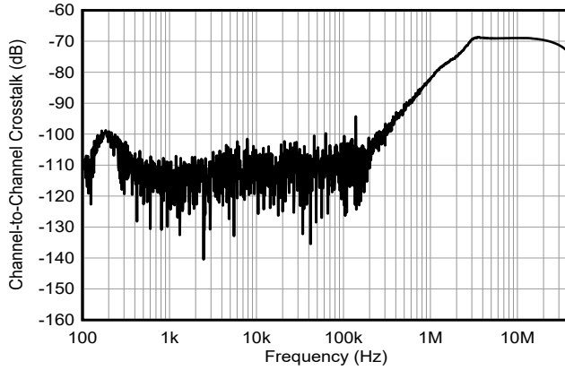
图 5-19. 通道间串扰
