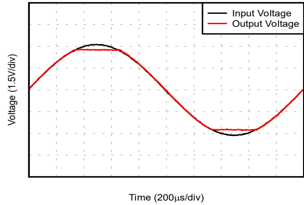
图 5-20. 无相位反转
