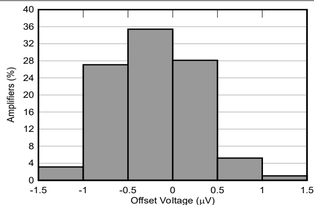
图 5-2. 失调电压分布图
