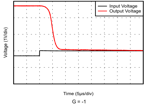
图 5-34. 过载恢复
