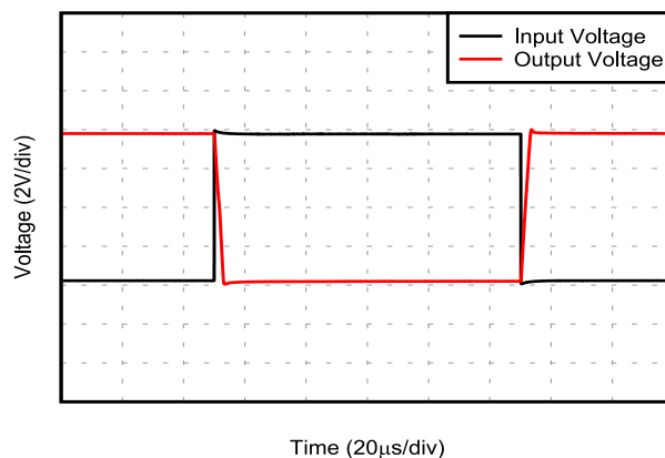
图 5-38. 大信号阶跃响应
