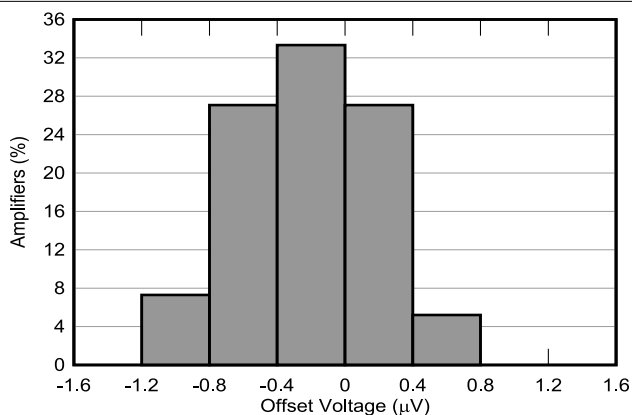
图 5-1. 失调电压分布图
