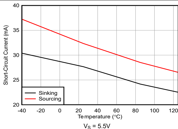
图 5-29. 短路电流与温度间的关系
