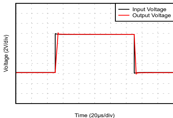
图 5-37. 大信号阶跃响应
