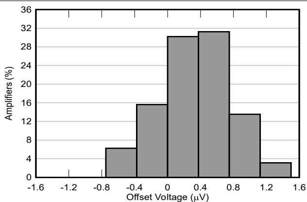
图 5-1. 失调电压分布图
