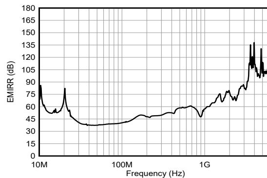
图 6-2. EMI 抑制比
