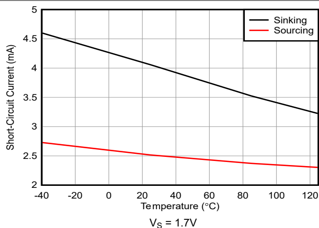
图 5-30. 短路电流与温度间的关系
