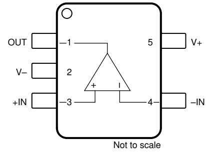
图 4-2. OPA237 : DBV 封装, 5 引脚 SOT-23 (顶视图)
