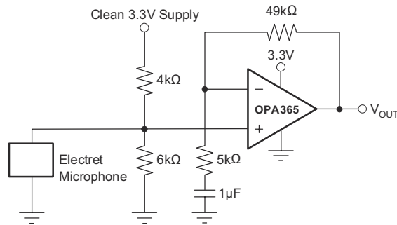
图 9-2. 麦克风前置放大器
