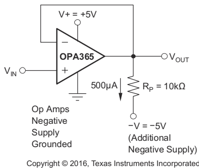
图 8-4. 摆动到接地
