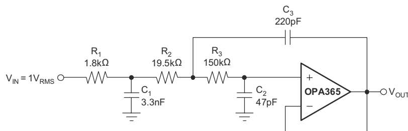
图 8-6. 配置为三级 20kHz Sallen-Key 滤波器
