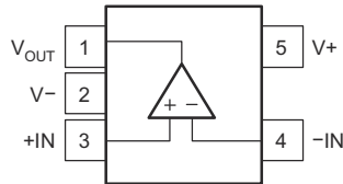
图 6-1. OPA365 : DBV 封装, 5 引脚 SOT-23 ( 顶视图 )
