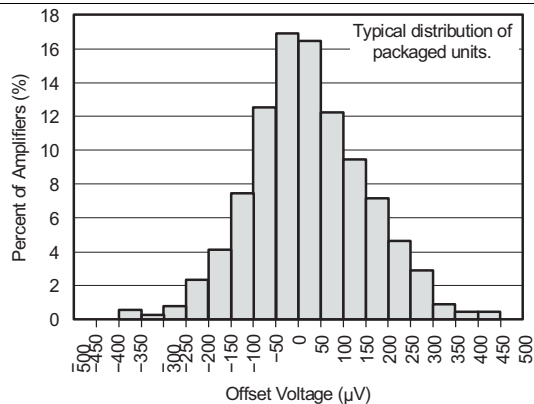
图 19. 失调电压产生分布
