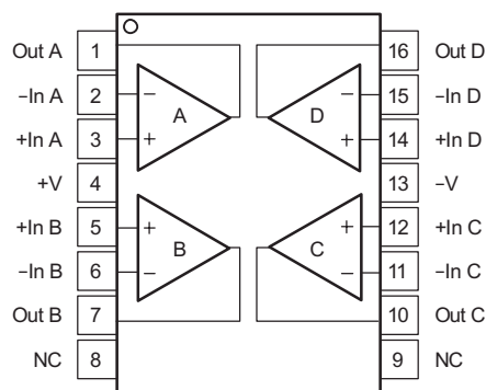
DBQ 封装 16 引脚 SSOP 俯视图
