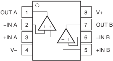
图 4-3. OPA2328 D 封装，8 引脚 SOIC 和 DGK 封装，8 引脚 VSSOP (顶视图)
