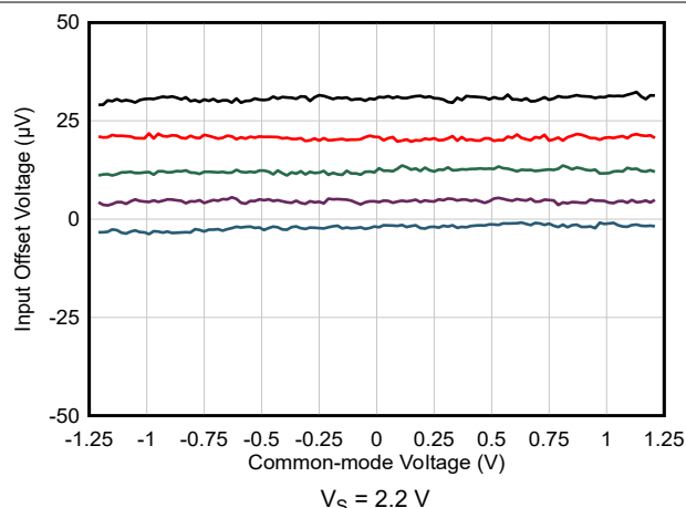
图 5-3. 失调电压与共模电压间的关系
