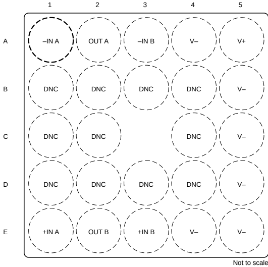
图 4-5. OPA2328 YBJ 封装，24 引脚 DSBGA (顶视图)
