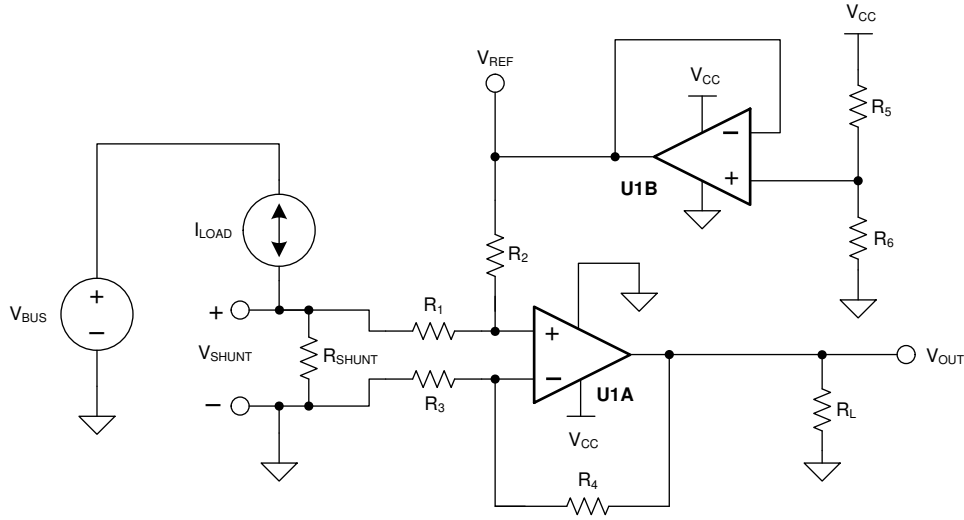
图 7-2. 双向电流检测原理图
