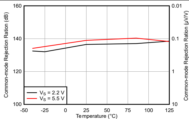
图 5-14. CMRR 与温度间的关系
