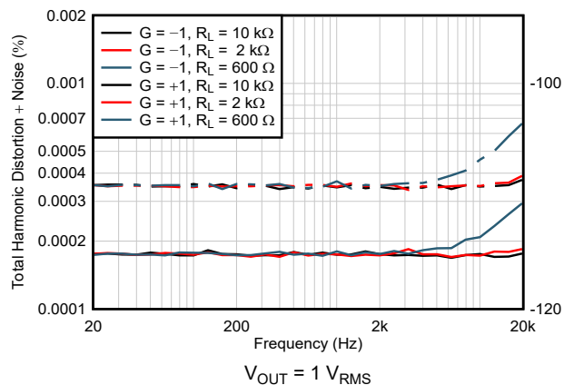
图 5-30. THD+N 与频率间的关系
