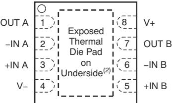
图 4-4. OPA2328 DRG 封装，8 引脚 WSON (顶视图)
