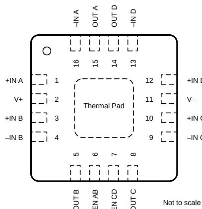
图 4-7. OPA4328 RUM 封装 ( 预发布 ) , 16 引脚 WQFN ( 顶视图 )
