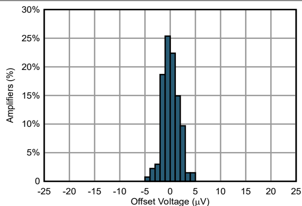
图 5-2. 失调电压生产分配
