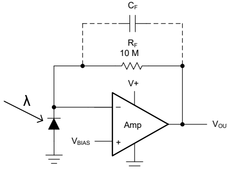
图 7-5. 单电源跨导放大器
