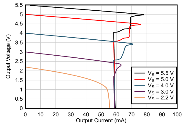
图 5-21. 输出电压摆幅与输出电流间的关系
