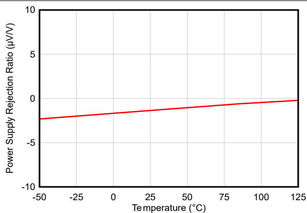
图 5-13. PSRR 与温度间的关系
