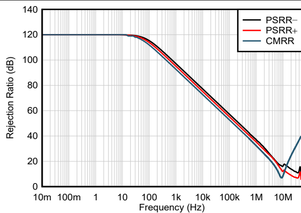
图 5-15. CMRR 和 PSRR 与频率间的关系
