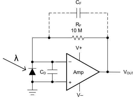
图 7-4. 双电源跨导放大器
