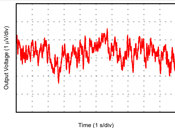
图 5-17. 0.1Hz 至 10Hz 输入电压噪声
