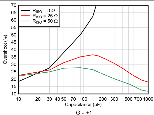
图 5-28. 小信号过冲与负载电容间的关系
