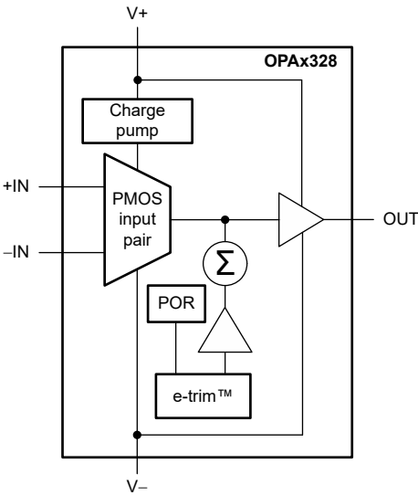
方框图
