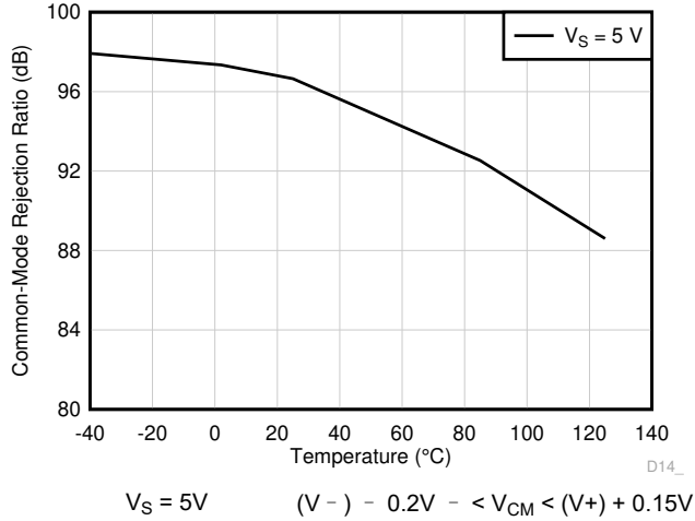
图 6-33. 直流 CMRR 与温度间的关系
