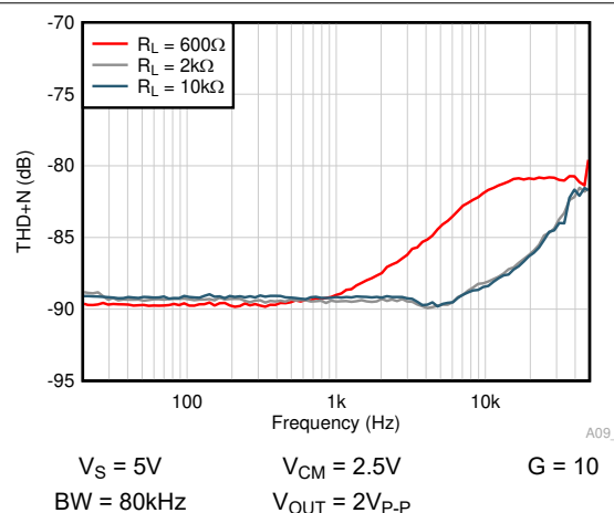
图 6-38. THD+N 与频率间的关系
