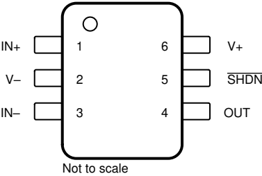
图 5-4. OPA323S DCK 封装， 6 引脚 SC70 (顶视图)
