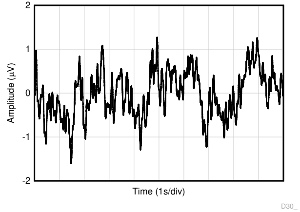
图 6-34. 0.1Hz 至 10Hz 时域电压噪声
