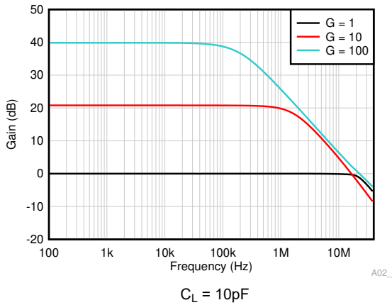
图 6-21. 闭环增益与频率间的关系
