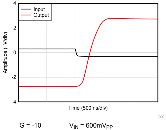
图 6-57. 过载恢复
