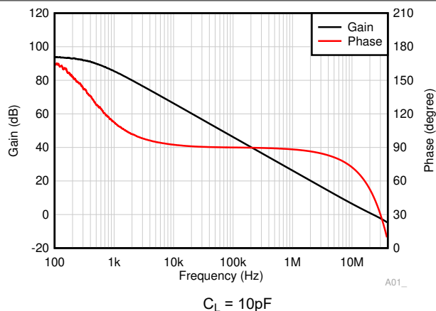
图 6-19. 开环增益和相位与频率间的关系
