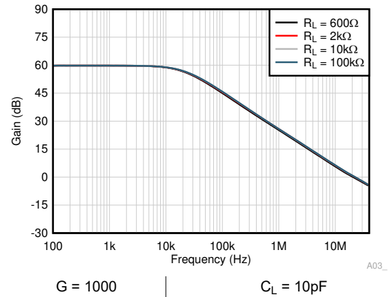
图 6-22. 闭环增益与频率间的关系
