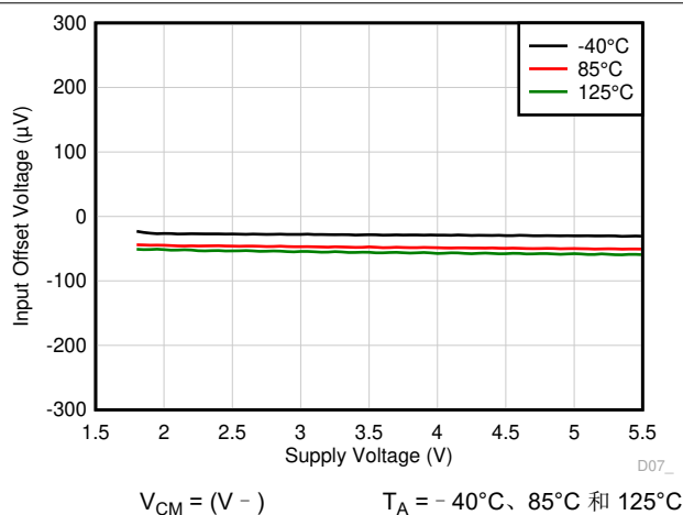
图 6-8. 输入失调电压与电源电压间的关系
