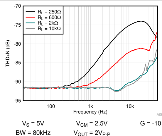
图 6-39. THD+N 与频率间的关系
