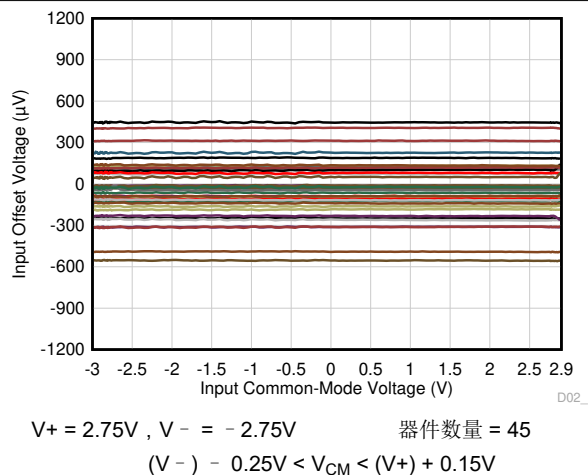
图 6-10. 输入偏移偏置电压与共模
