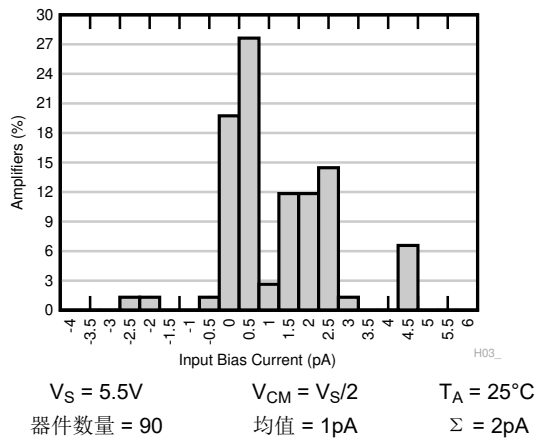
图 6-3. 输入偏置电流分布直方图
