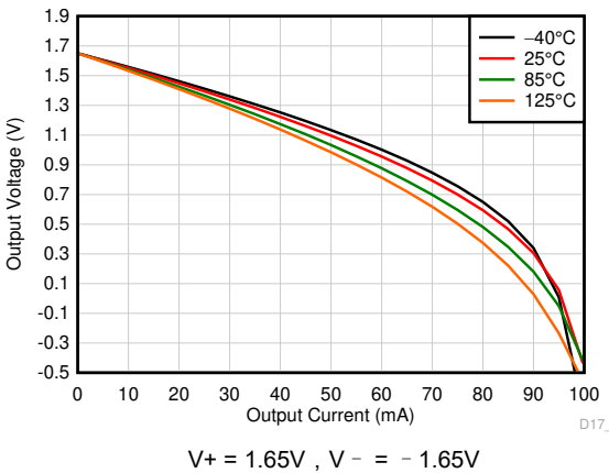
图 6-25. 输出电压摆幅与输出电流 (拉电流) 间的关系
