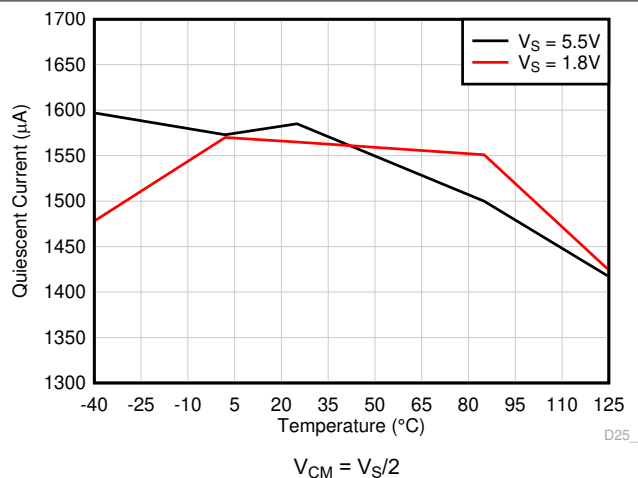
图 6-52. 静态电流与温度间的关系
