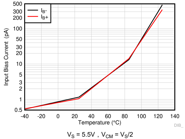
图 6-14. I_B 与温度间的关系
