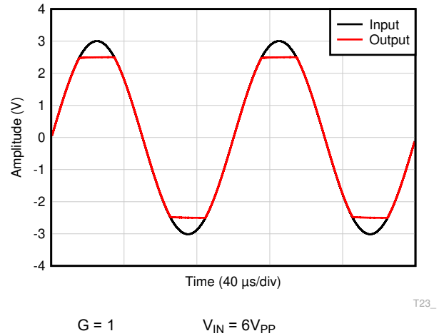
图 6-56. 无相位反转
