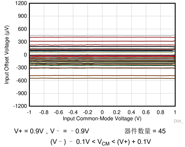
图 6-12. 输入偏移偏置电压与共模
