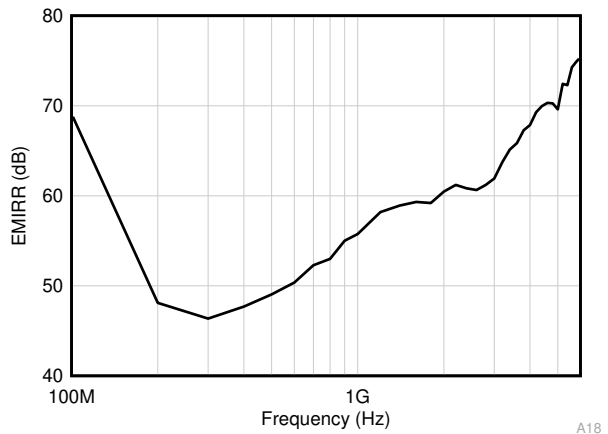
图 6-69. 以同相输入为基准的电磁干扰抑制比 (EMIRR+) 与频率间的关系
