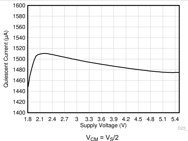
图 6-50. 静态电流与电源电压间的关系
