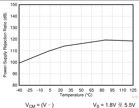
图 6-31. 直流 PSRR 与温度间的关系
