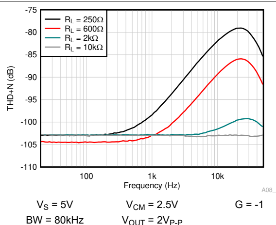
图 6-37. THD+N 与频率间的关系
