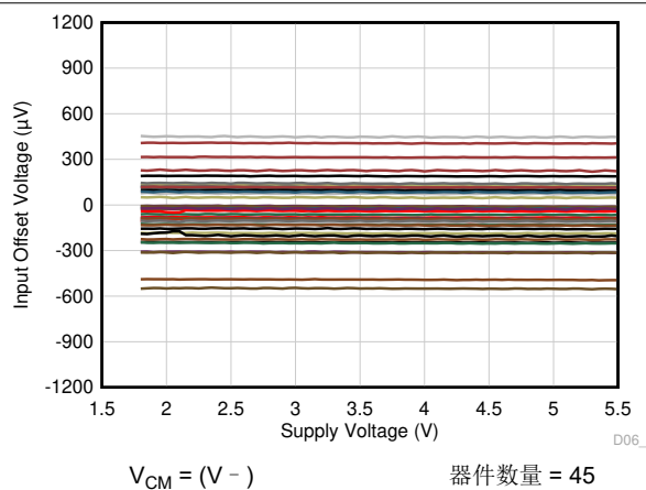
图 6-7. 输入失调电压与电源电压间的关系
