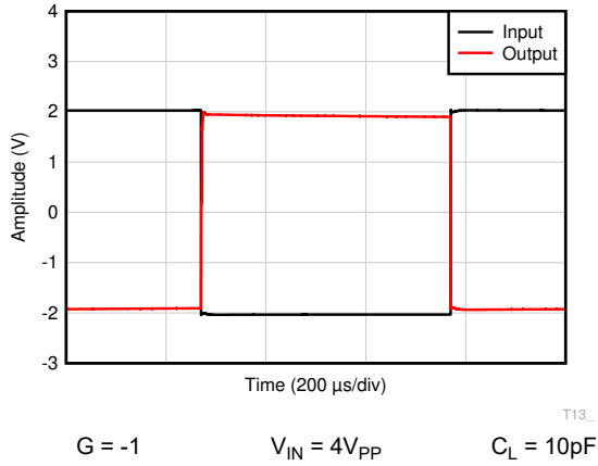
图 6-65. 大信号阶跃响应
