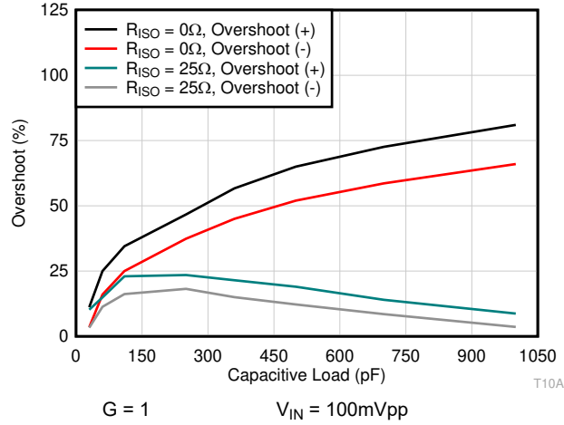
图 6-53. 小信号过冲与容性负载间的关系
