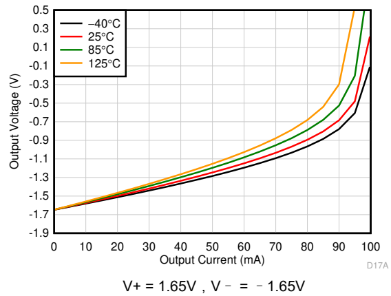
图 6-26. 输出电压摆幅与输出电流 (灌电流) 间的关系
