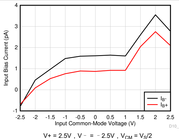
图 6-16. I_B 与共模电压间的关系
