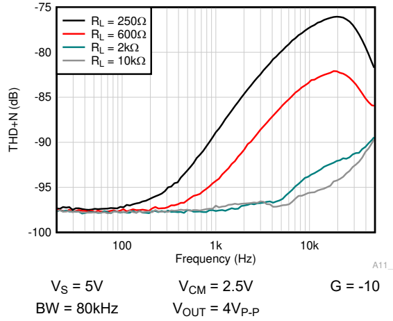
图 6-43. THD+N 与频率间的关系
