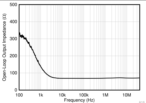
图 6-20. 开环输出阻抗与频率间的关系
