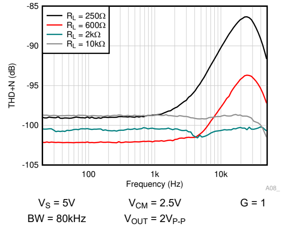
图 6-36. THD+N 与频率间的关系
