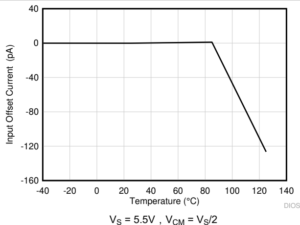
图 6-15. I_{OS} 与温度间的关系
