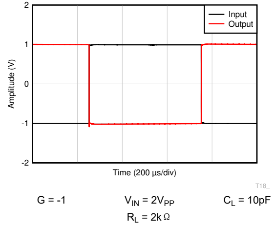
图 6-66. 大信号阶跃响应
