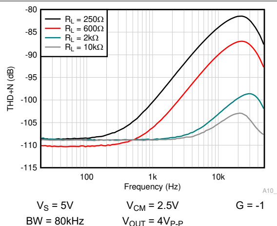
图 6-41. THD+N 与频率间的关系
