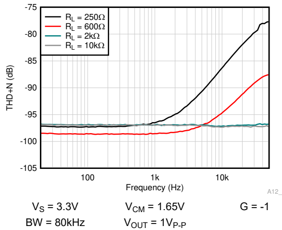
图 6-47. THD+N 与频率间的关系
