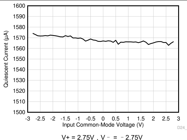
图 6-51. 静态电流与共模电压间的关系
