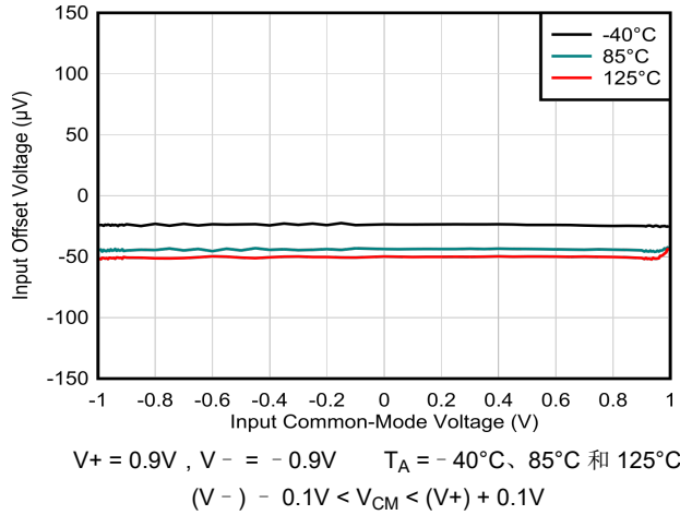
图 6-13. 输入偏移偏置电压与共模
