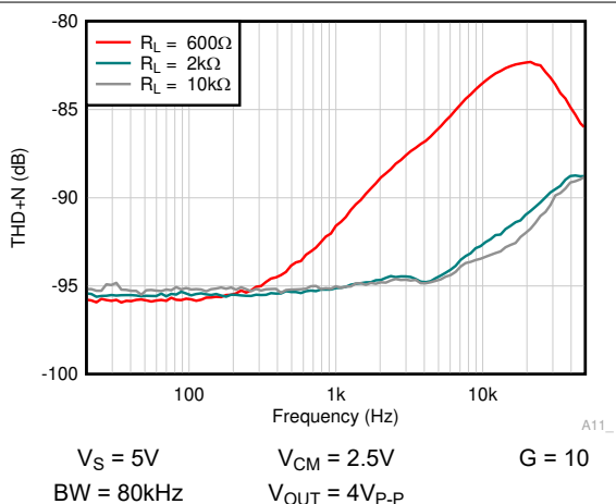
图 6-42. THD+N 与频率间的关系
