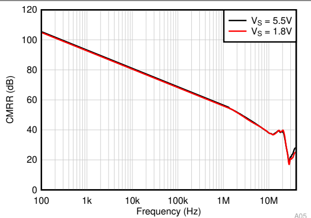
图 6-32. CMRR 与频率间的关系
