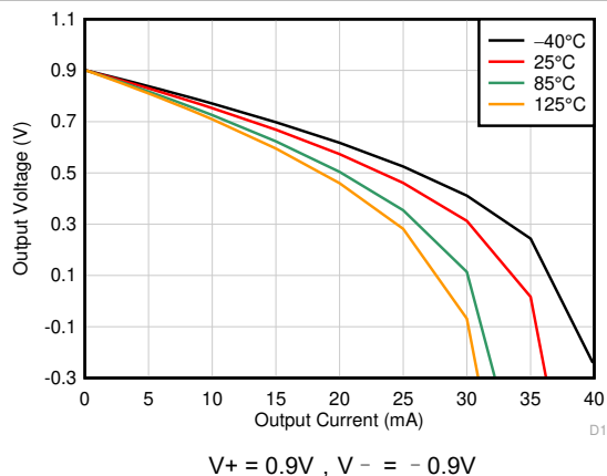
图 6-27. 输出电压摆幅与输出电流 (拉电流) 间的关系
