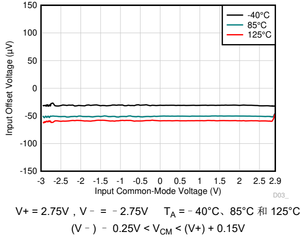
图 6-11. 输入偏移偏置电压与共模
