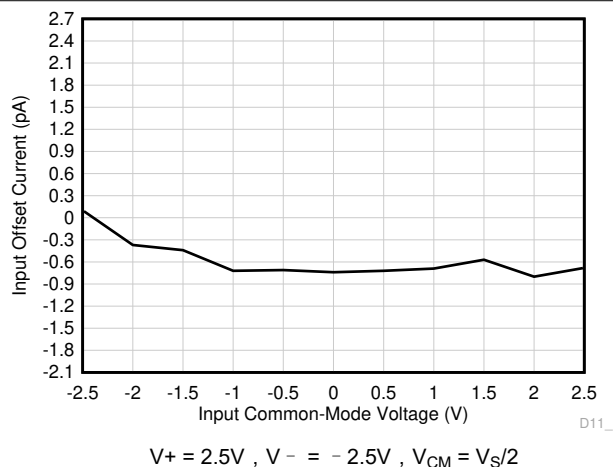
图 6-17. I_{OS} 与共模电压间的关系
