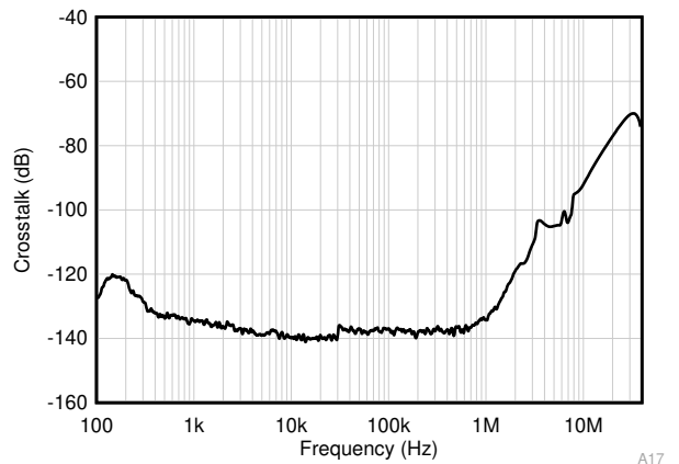
图 6-70. 通道隔离
