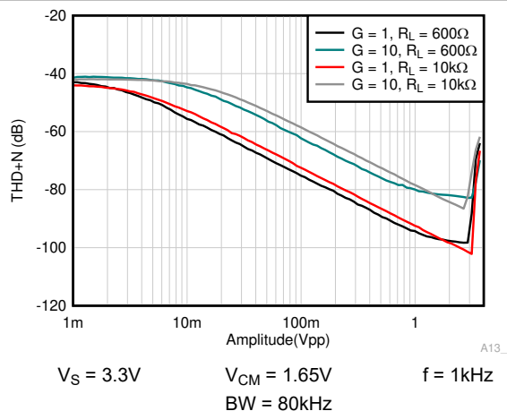
图 6-49. THD + N 与幅度间的关系
