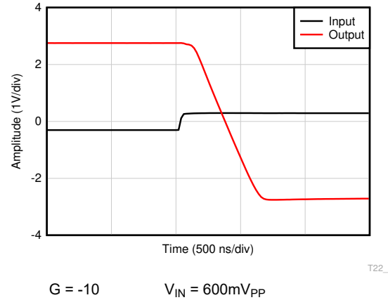
图 6-58. 过载恢复
