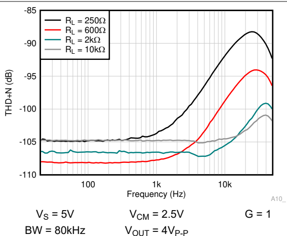
图 6-40. THD+N 与频率间的关系
