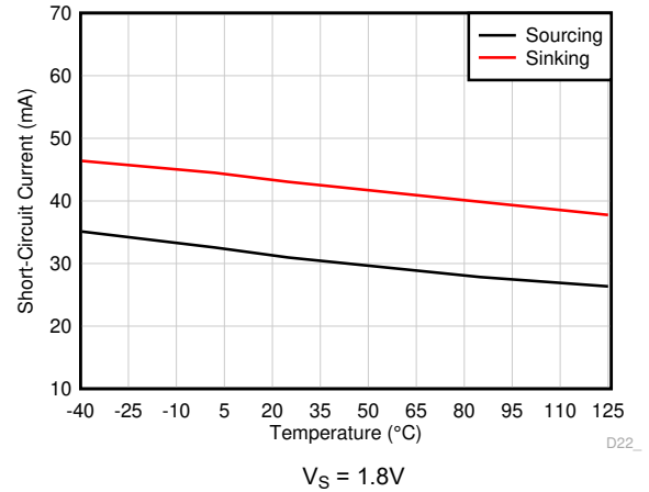
图 6-68. 短路电流与温度间的关系
