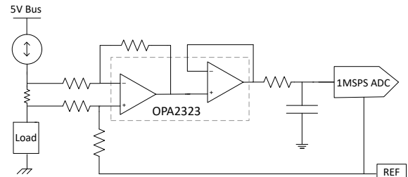
双向高侧电流检测放大器和 ADC 驱动器
