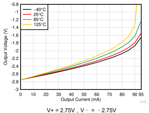
图 6-24. 输出电压摆幅与输出电流 (灌电流) 间的关系
