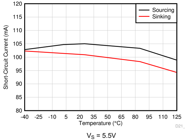
图 6-67. 短路电流与温度间的关系
