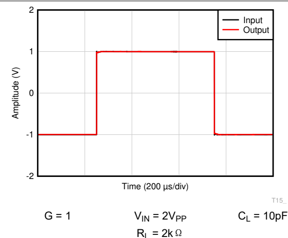
图 6-64. 大信号阶跃响应
