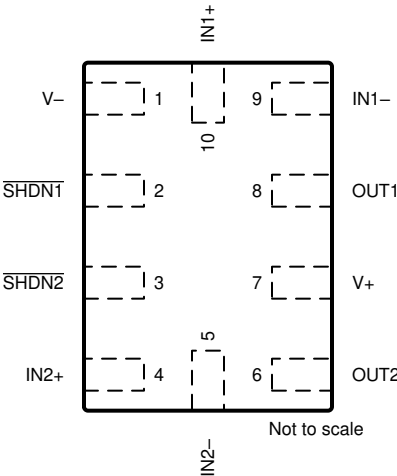
图 5-7. OPA2323S RUG 封装 10 引脚 X2QFN ( 顶视图 )
