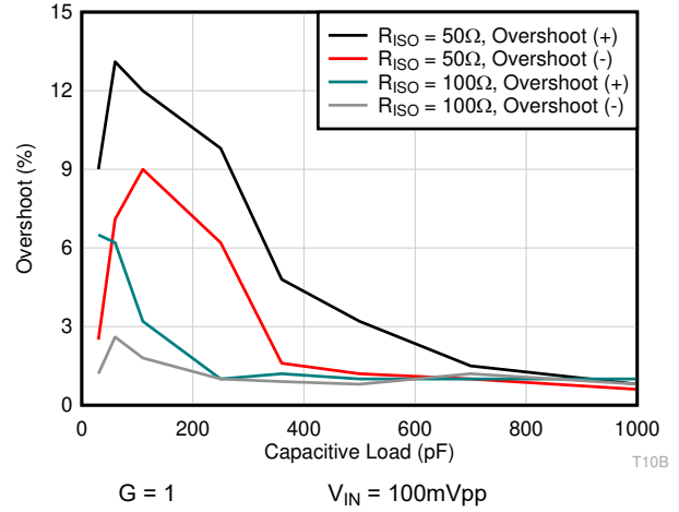
图 6-54. 小信号过冲与容性负载间的关系
