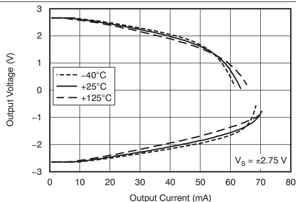
图 14. 输出电压摆幅与输出电流间的关系
