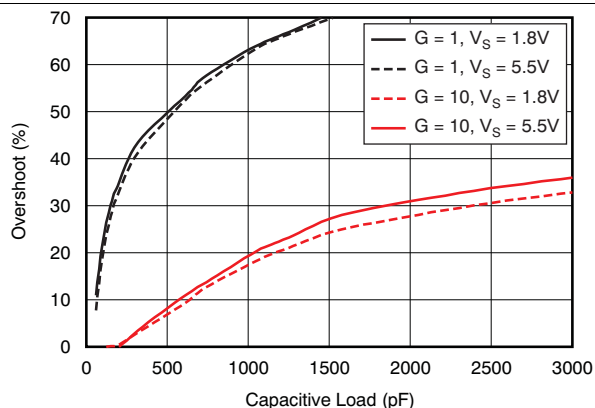
图 20. 小信号过冲与负载电容间的关系
