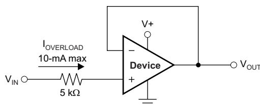
图 33. 输入电流保护
