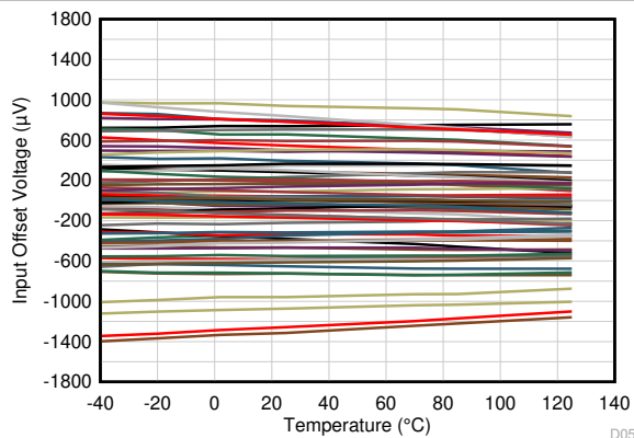
图 6-8. 输入失调电压与温度间的关系
