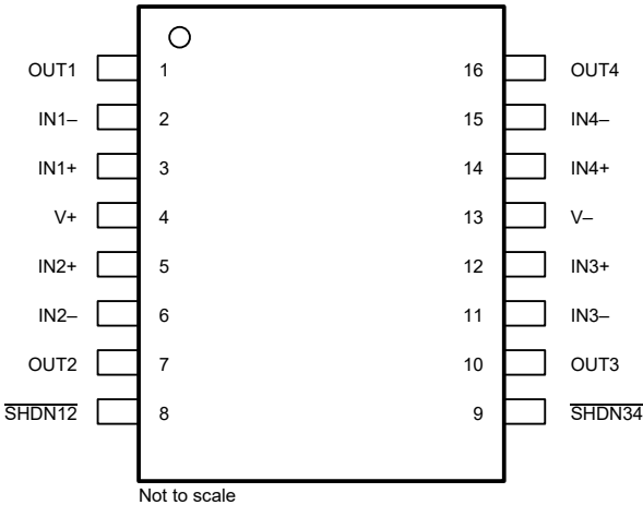
图 5-13. OPA4310S DYY 封装， 16 引脚 SOT-23-THIN ( 顶视图 )
