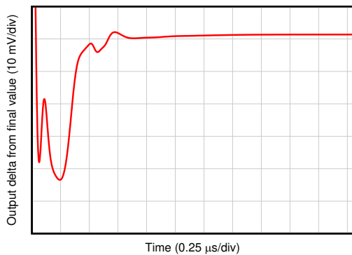
图 6-45. 小信号阶跃响应
