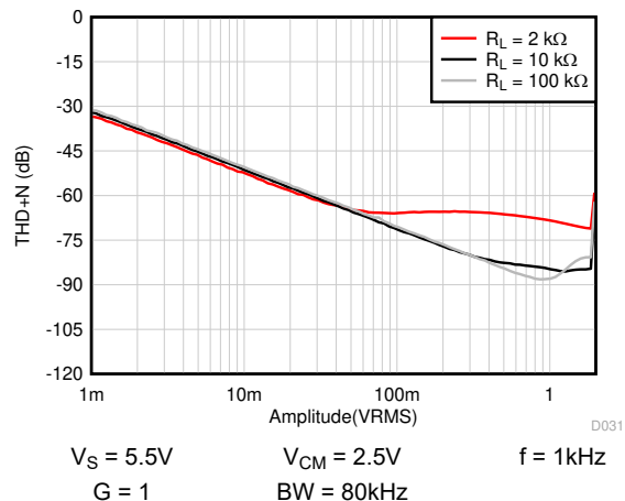
图 6-33. THD + N 与幅度间的关系
