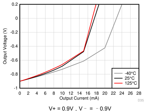
图 6-24. 输出电压摆幅与输出电流 (灌电流) 间的关系
