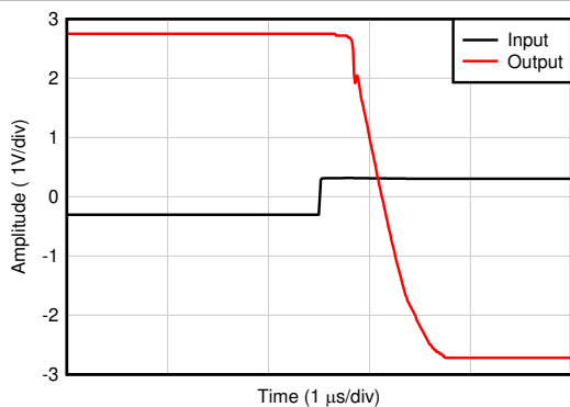
图 6-43. 过载恢复
