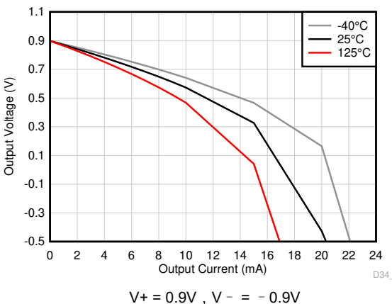
图 6-23. 输出电压摆幅与输出电流 (拉电流) 间的关系
