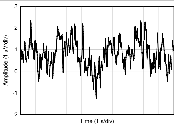
图 6-29. 0.1Hz 至 10Hz 时域电压噪声
