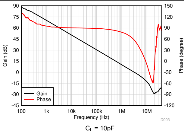
C_L = 10\text{pF} 图 6-18. 开环增益和相位与频率间的关系
