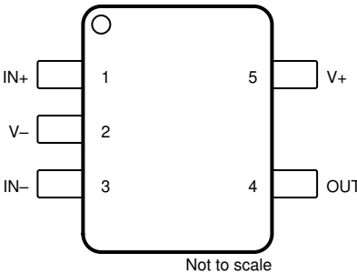
图 5-2. OPA310 DCK 和 DRL 封装， 5 引脚 SC70 和 5 引脚 SOT-5X3 (顶视图)
