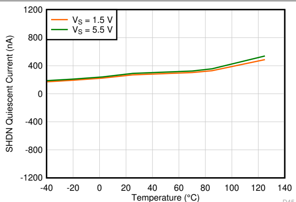
图 6-53. 关断模式静态电流与温度间的关系
