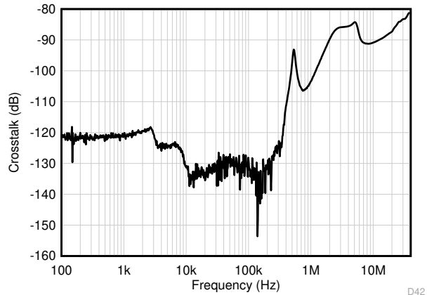
图 6-57. 通道隔离
