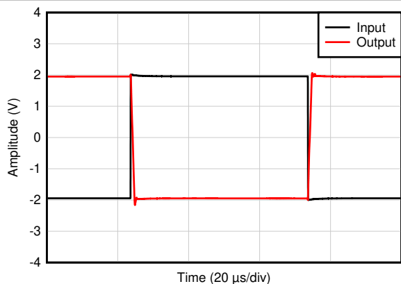
图 6-49. 大信号阶跃响应
