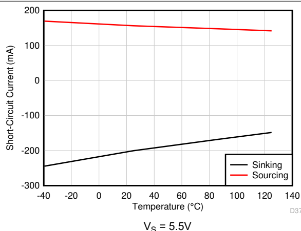
图 6-51. 短路电流与温度间的关系
