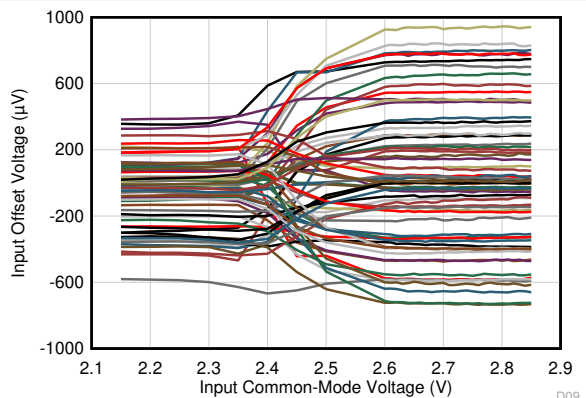
图 6-9. 失调电压与共模间的关系
