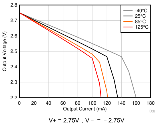
图 6-21. 输出电压摆幅与输出电流 (拉电流) 间的关系
