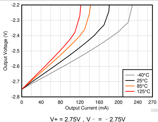
图 6-22. 输出电压摆幅与输出电流 (灌电流) 间的关系
