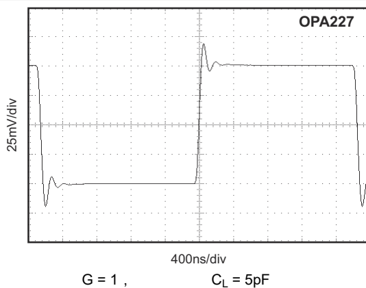
图 6-29. 小信号阶跃响应
