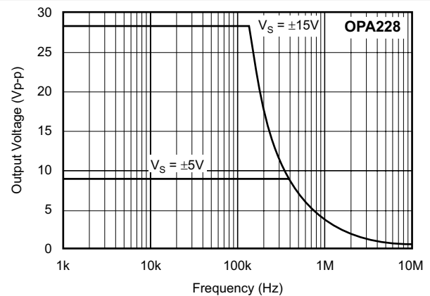
图 6-30. 最大输出电压与频率间的关系
