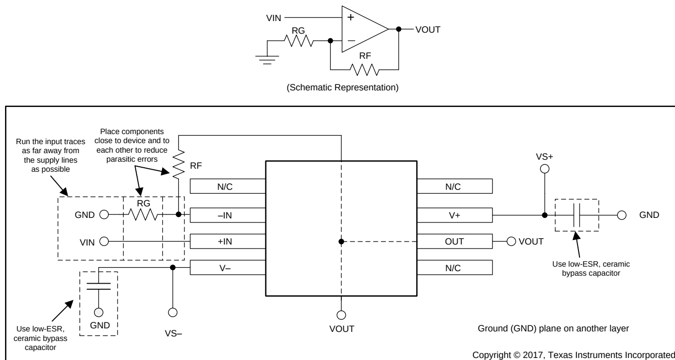
图 50. 布局示例
