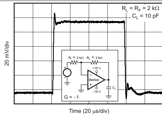
图 28. 负过载恢复
