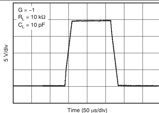
图 32. 大信号阶跃响应
