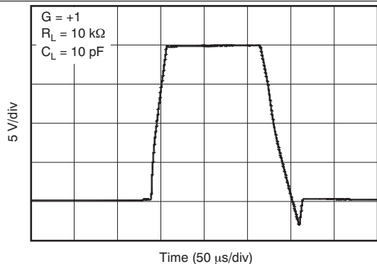
图 31. 大信号阶跃响应
