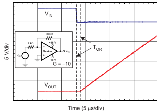
图 26. 无相位反转
