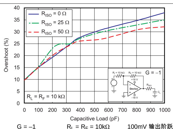
图 41. 小信号过冲与容性负载间的关系
