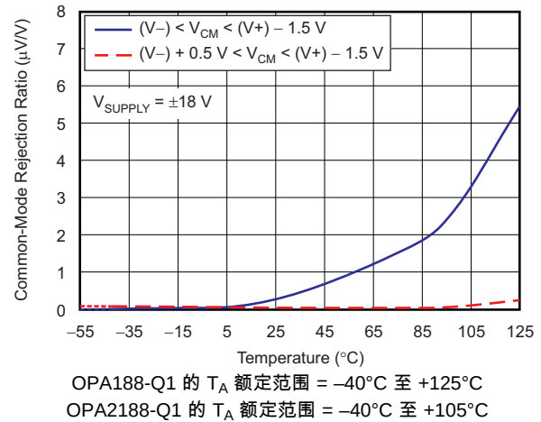
图 14. CMRR 与温度间的关系
