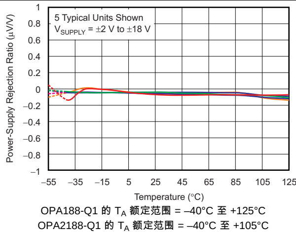
图 15. PSRR 与温度间的关系
