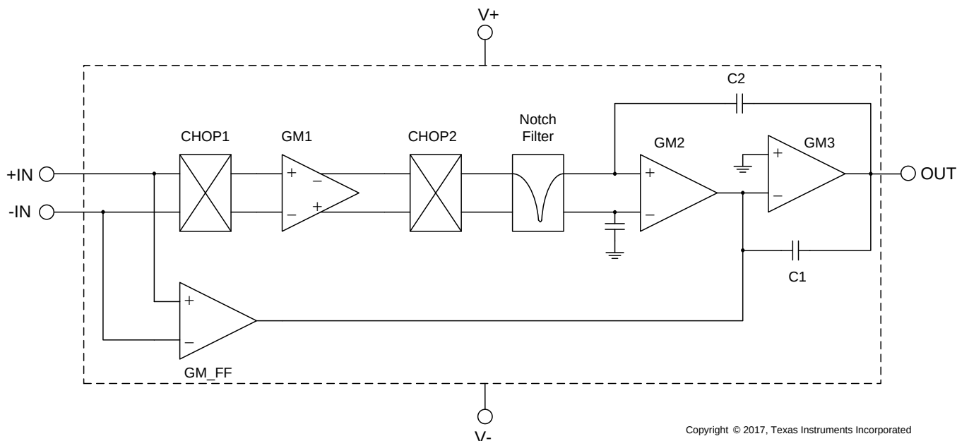
图 37. 功能框图
