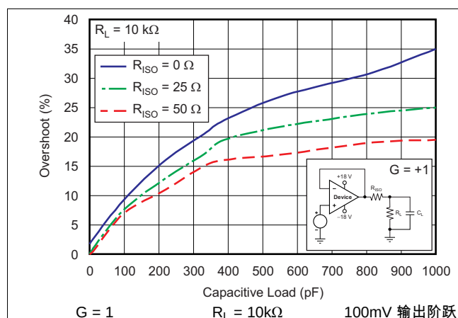
图 40. 小信号过冲与容性负载间的关系
