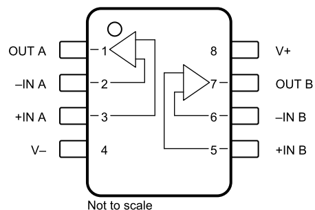
引脚功能
