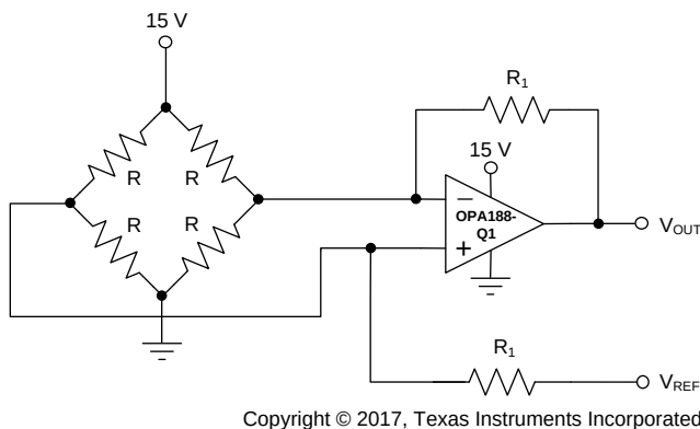
图 46. 桥式放大器
