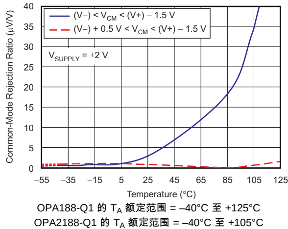
图 13. CMRR 与温度间的关系
