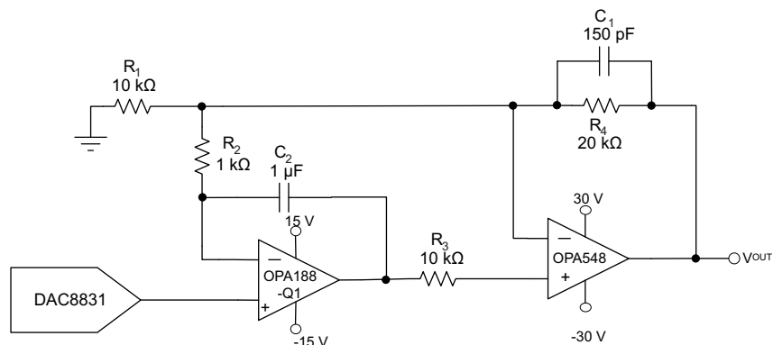
图 48. 可编程电源
