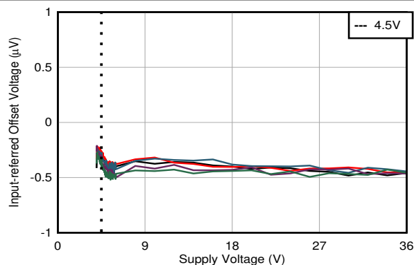
图 7-7. 偏移电压与电源电压间的关系
