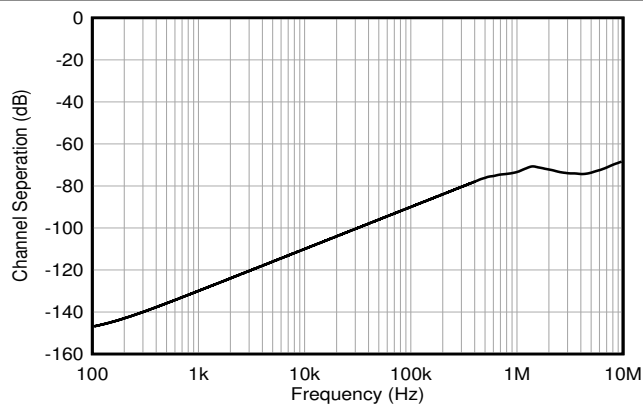
图 7-38. 通道分离
