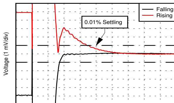
图 7-32. 大信号阶跃响应
