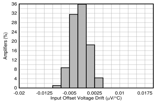
图 7-2. 失调电压漂移分配
