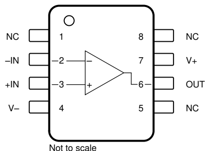
图 6-1. OPA182 D ( 8 引脚 SOIC ) 封装，顶视图
