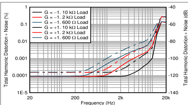
图 7-19. THD+N 比与频率间的关系
