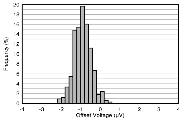
图 7-1. 失调电压生产分配
