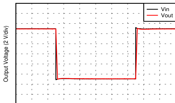
图 7-31. 小信号阶跃响应
