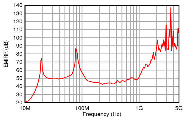
图 7-37. EMIRR 与频率之间的关系
