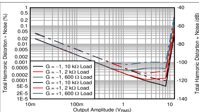
图 7-20. THD+N 与输出幅度间的关系
