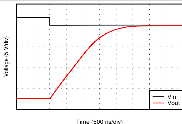
图 7-27. 无相位反转
