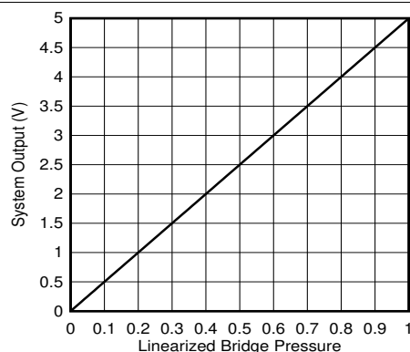
图 9-4. 电桥输出
