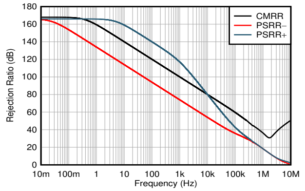
图 7-14. CMRR 和 PSRR 与频率间的关系
