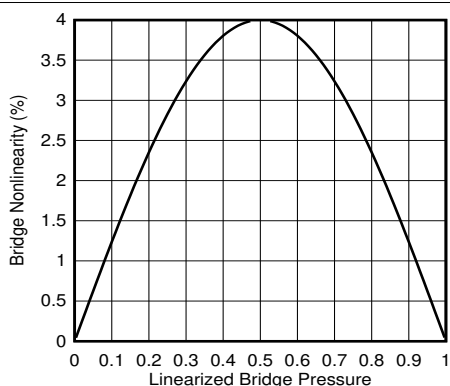
图 9-3. 电桥非线性
