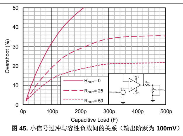
图 44. 小信号过冲与容性负载间的关系（输出阶跃为 100mV）
