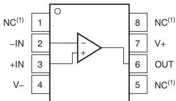
图 4-3. OPA171 D 封装：8 引脚 SOIC（顶视图）
