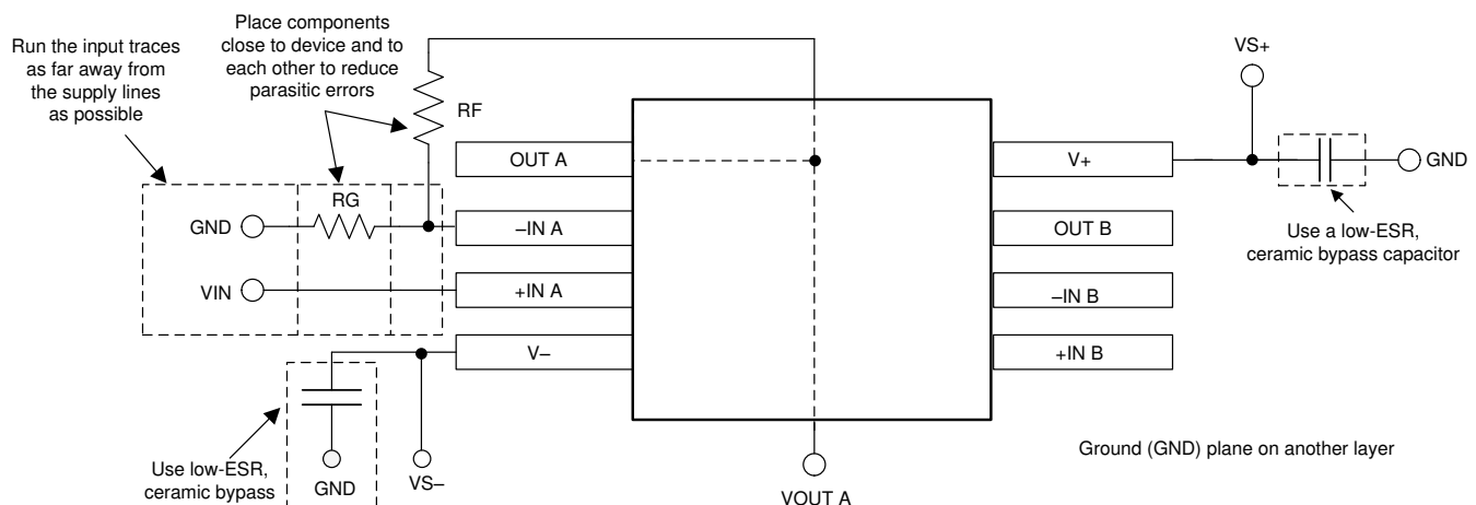
图 10-1. OPA2210 Layout Example
