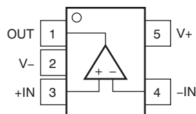
OPA188 DBV 封装 5 引脚 SOT-23 俯视图
