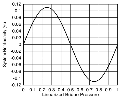
图 9-5. 系统非线性
