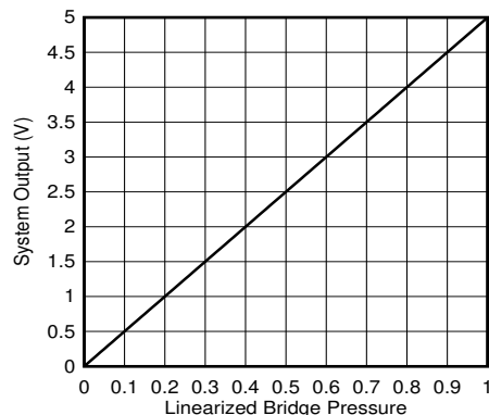
图 9-4. 电桥输出
