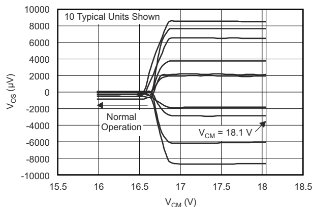
图 6-5. 失调电压与共模电压间的关系: V_{\text{SUPPLY}} (\text{V}) = \pm 18\text{V} (前级)
