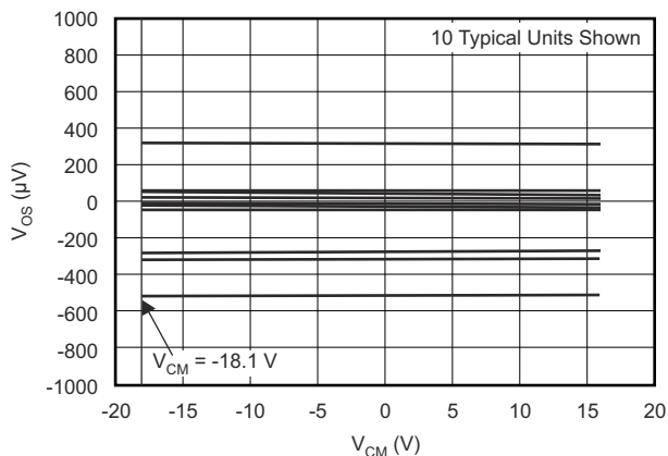
图 6-4. 失调电压与共模电压间的关系: V_{\text{SUPPLY}} (\text{V}) = \pm 18\text{V}
