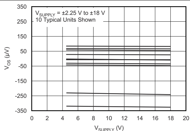
图 5-6. 失调电压与电源间的关系
