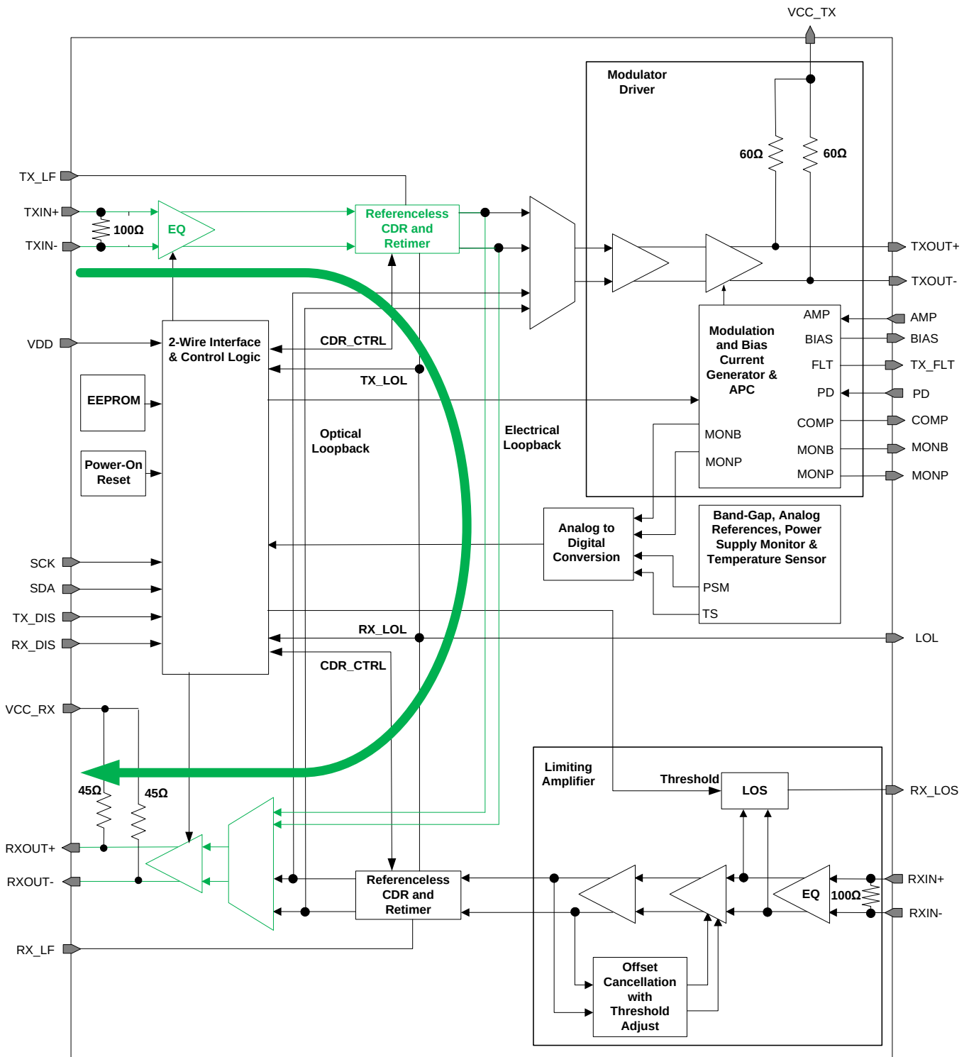
图 38. Electrical Loopback
