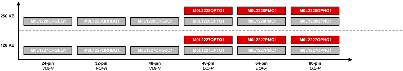
图 5-1. 器件比较图
