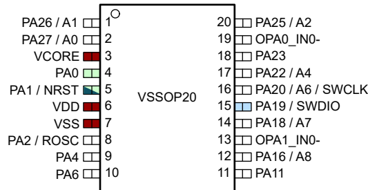
图 6-7. 20 引脚 DGS20 (VSSOP) (顶视图) - MSPM0L134x
