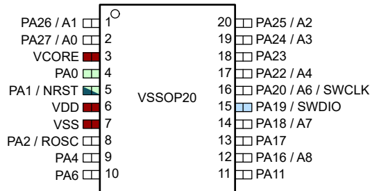
图 6-6. 20 引脚 DGS20 (VSSOP) (顶视图) - MSPM0L130x
