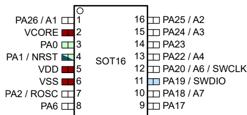
图 6-9. 16 引脚 DYY (SOT) (顶视图) - MSPM0L130x
