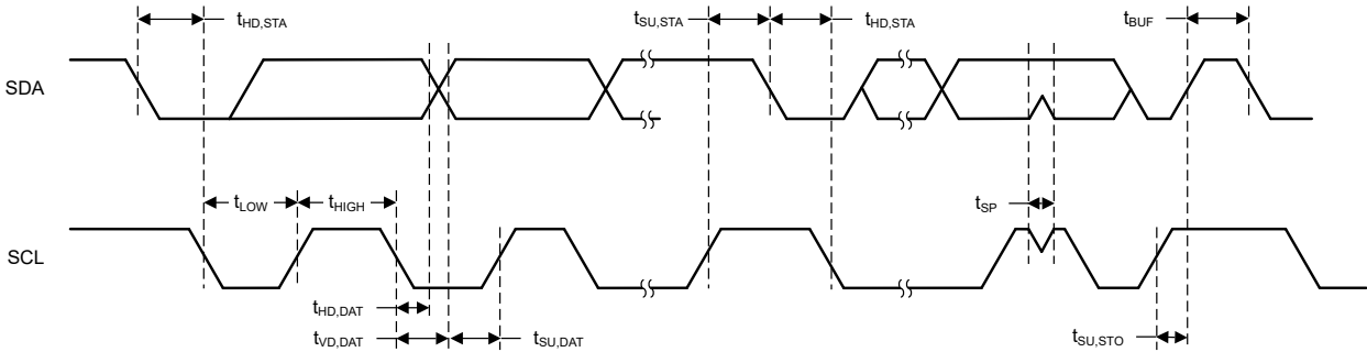
图 7-4. I2C 时序图
