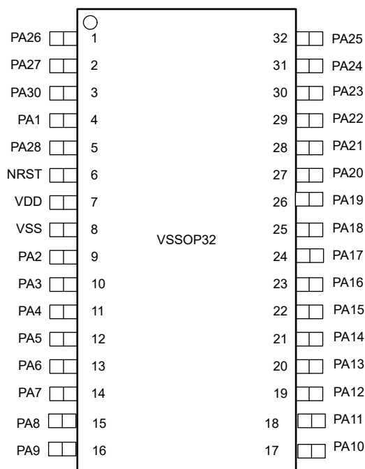
图 6-6. 32 引脚 DGS32 (VSSOP) ( 顶视图 )
