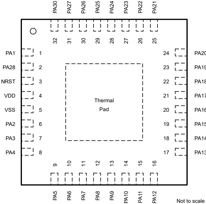
图 6-5. 32 引脚 RHB (VQFN) ( 顶视图 )
