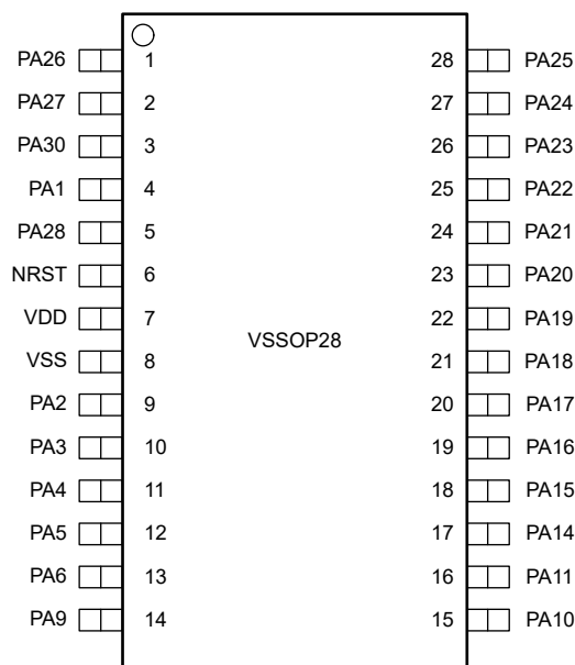
图 6-7. 28 引脚 DGS28 (VSSOP) ( 顶视图 )
