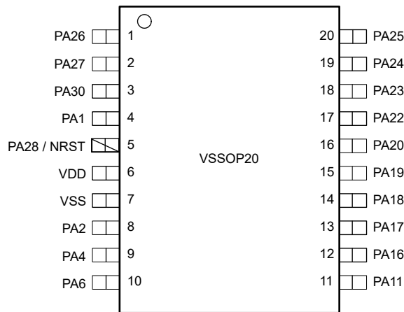
图 6-9. 20 引脚 DGS20 (VSSOP) (顶视图)
