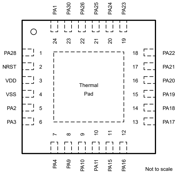
图 6-8. 24 引脚 RGE (VQFN) (顶视图)
