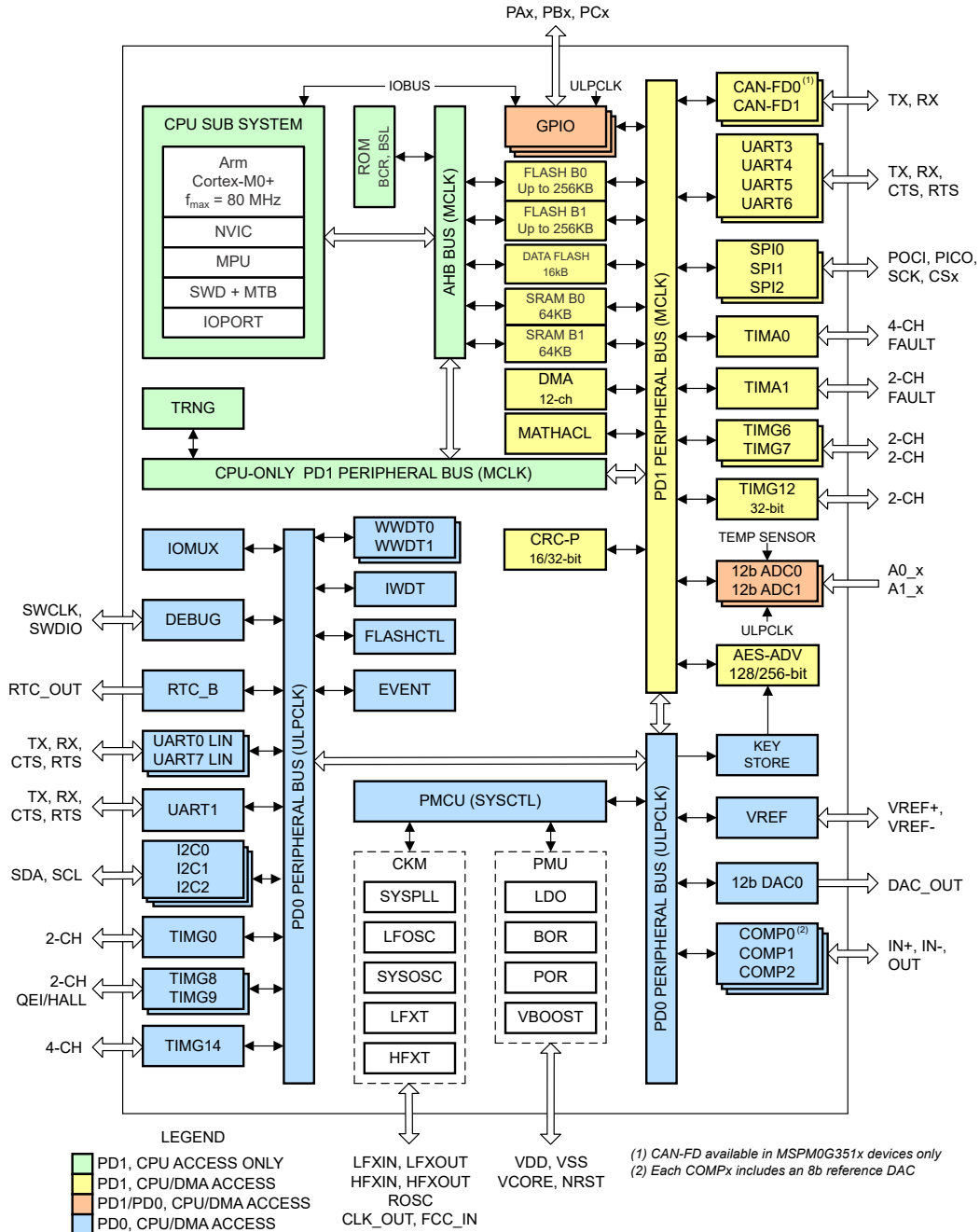
图 8-1. MSPM0G352x-Q1 功能方框图
