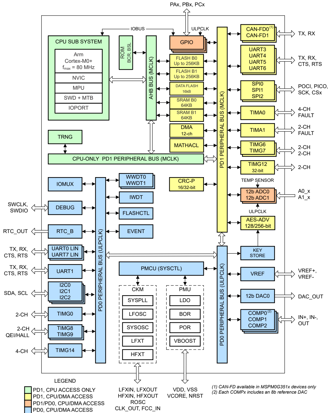
图 4-1. MSPM0G352x-Q1 功能方框图
