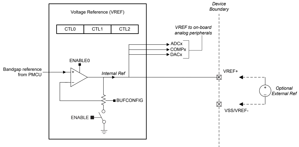
图 8-2. VREF 模块
