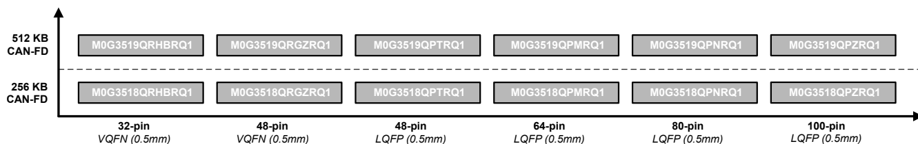
图 5-1. 器件比较图
