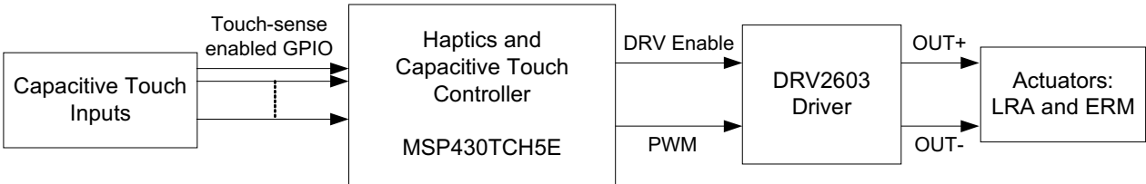
图 1. 独立应用，此类应用中，MSP430TCH5E 器件作为触觉和电容式触摸屏控制器
