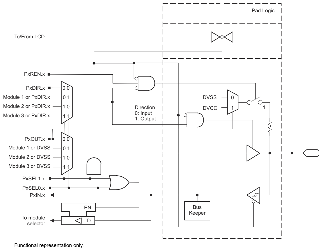
图 9-22. Port P6 (P6.4) Diagram
