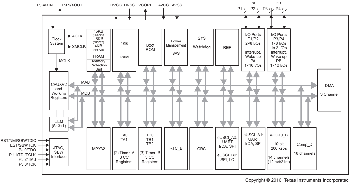
图 1-1. 功能方框图 - RHA 封装 - MSP430FR5721, MSP430FR5725, MSP430FR5729
