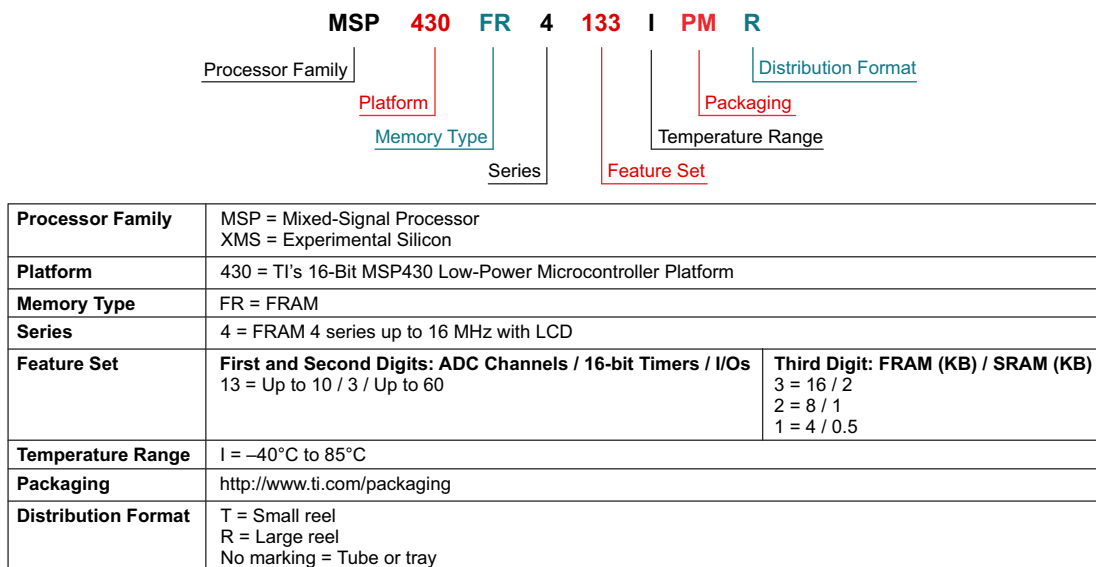
图 11-1. Device Nomenclature
