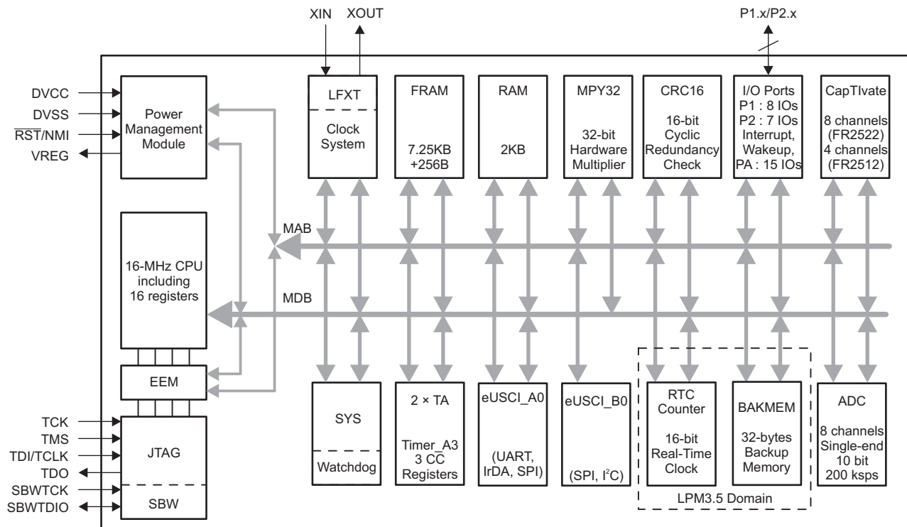
图 1-1. 功能框图
