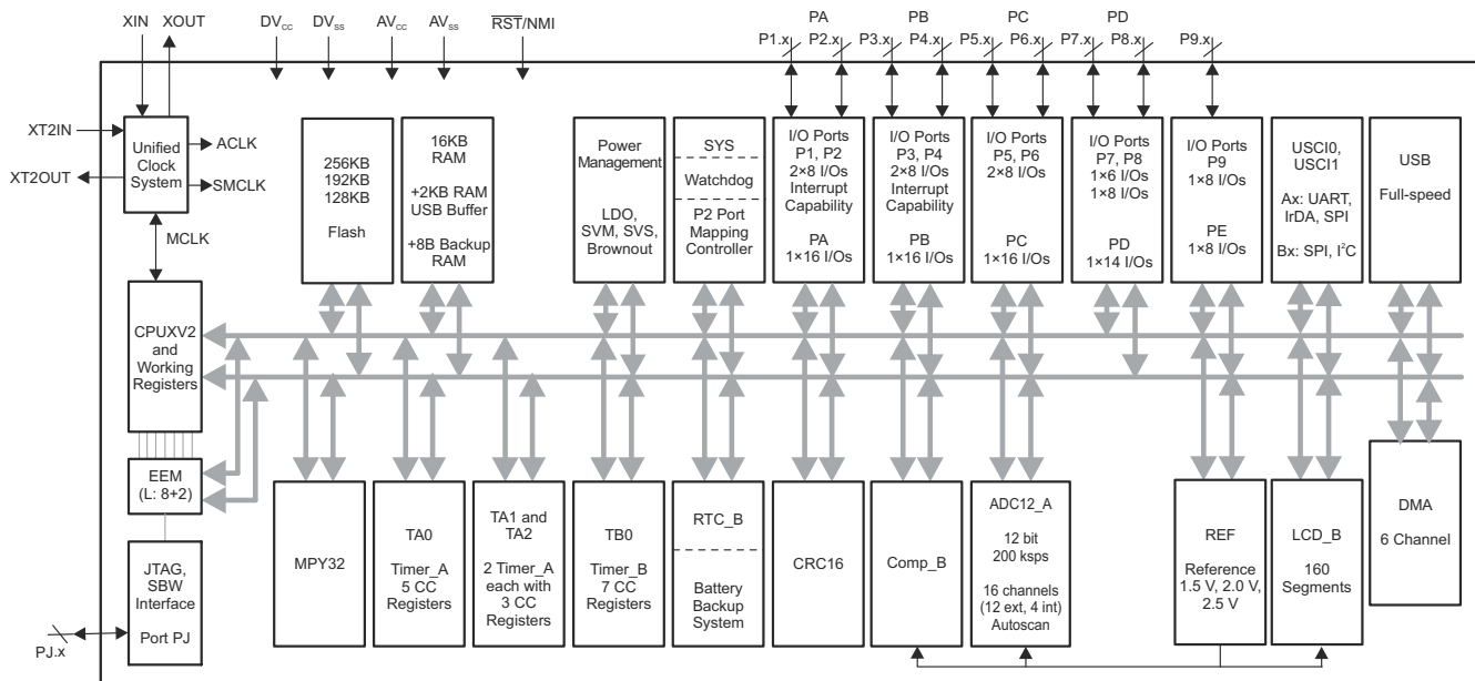
图 4-2. 功能框图 - MSP430F6635、MSP430F6634 和 MSP430F6633
