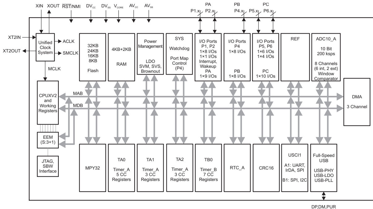
图 1-3. 功能方框图 - MSP430F5507IRGZ、MSP430F5506IRGZ、MSP430F5505IRGZ、MSP430F5504IRGZ、MSP430F5504IPT
