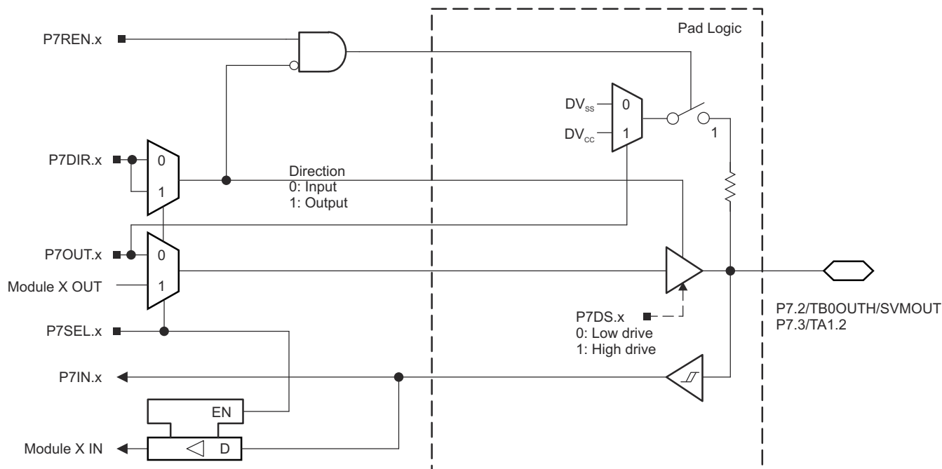
图 9-13. Port P7 (P7.2 and P7.3) Diagram
