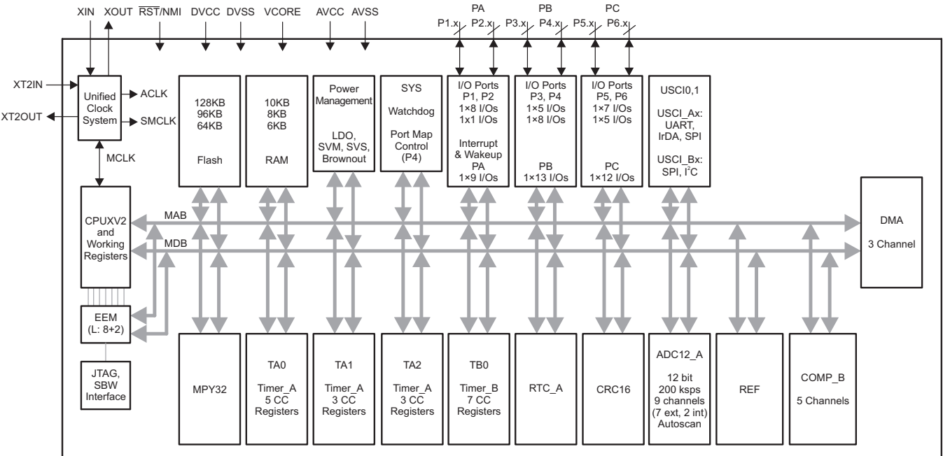
图 1-1. MSP430F534x 方框图
