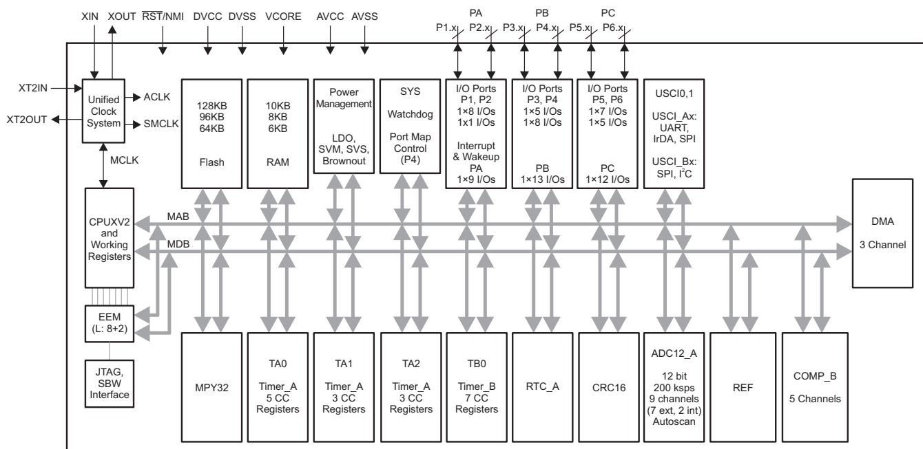
图 1-1. MSP430F534x 方框图
