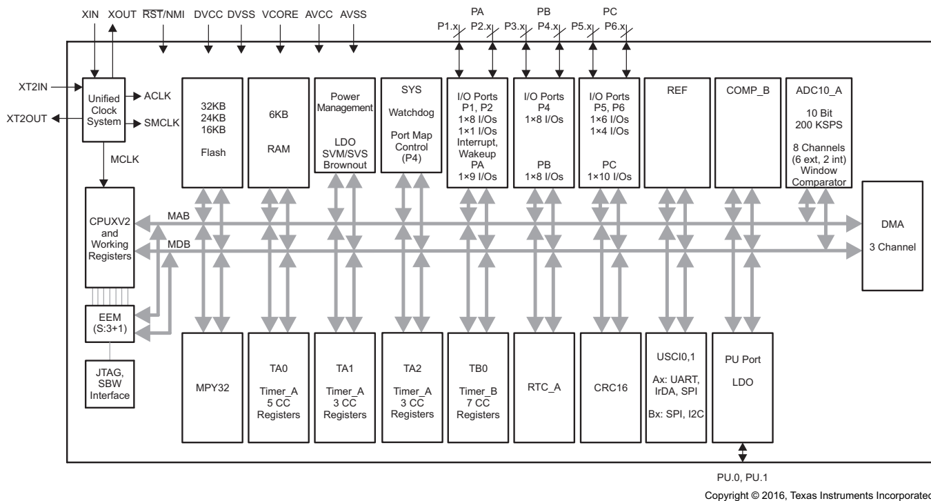
图 1-2. 功能方框图 – MSP430F5310IRGZ、MSP430F5309IRGZ、MSP430F5308IRGZ、MSP430F5310IPT、MSP430F5309IPT、MSP430F5308IPT
