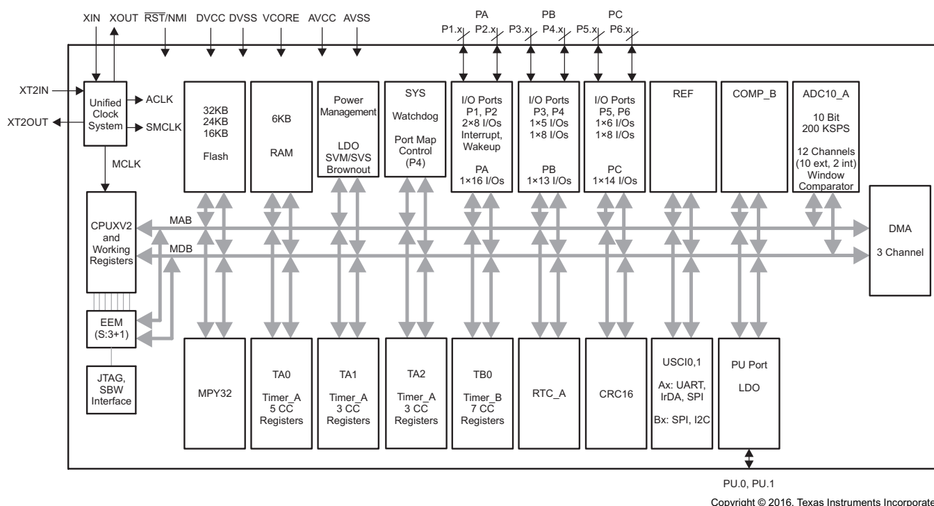
图 1-1. 功能方框图 – MSP430F5310IRGC、MSP430F5309IRGC、MSP430F5308IRG、MSP430F5310IZQE、MSP430F5309IZOE、MSP430F5308IZOE
