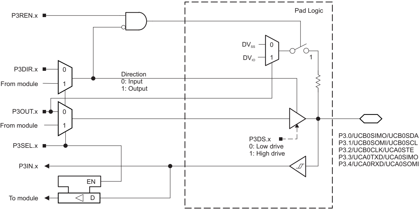
图 6-4. Port P3 (P3.0 to P3.4) Diagram
