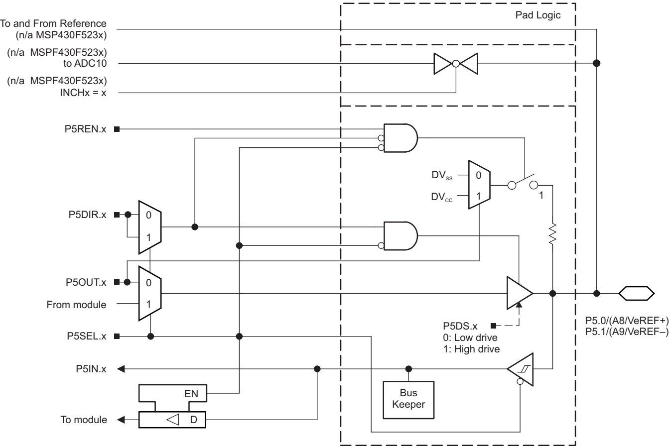
图 6-6. Port P5 (P5.0 and P5.1) Diagram
