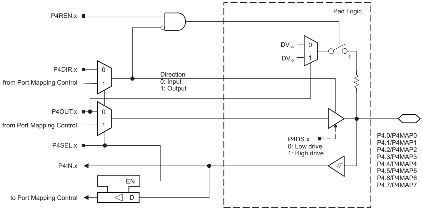
图 6-5. Port P4 (P4.0 to P4.7) Diagram
