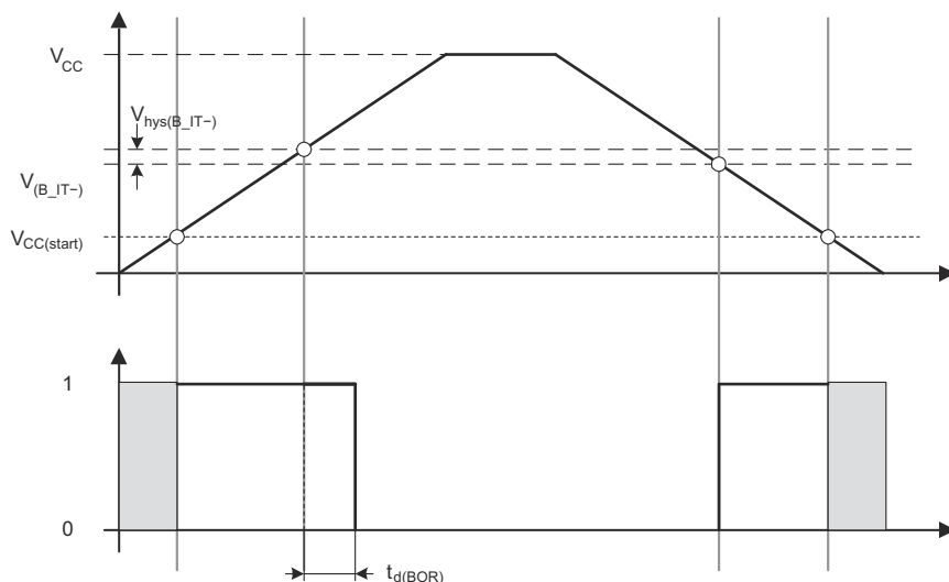
图 8-9. POR and BOR vs Supply Voltage
