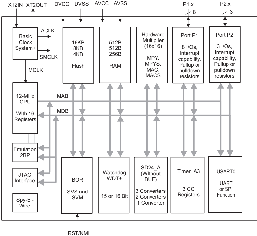
图 1-1. 功能框图
