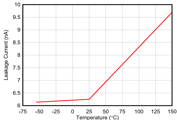
图 5-2. 漏电流与温度间的关系
