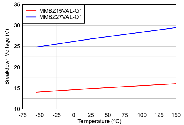
图 5-2. 击穿电压与温度间的关系
