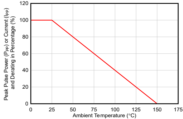
图 5-3. 峰值脉冲功率降额曲线
