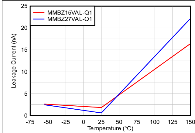
图 5-1. 漏电流与温度间的关系
