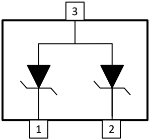
功能方框图
