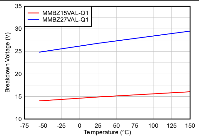
图 5-2. 击穿电压与温度间的关系
