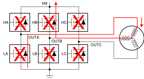
图 8-37. Coast State
