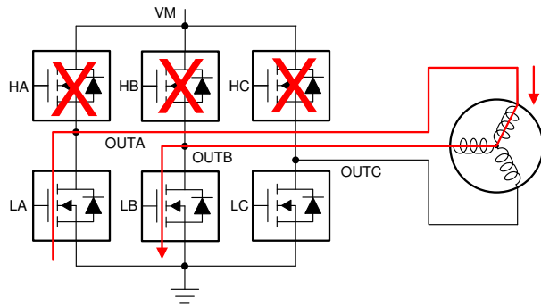
图 8-36. Brake State
