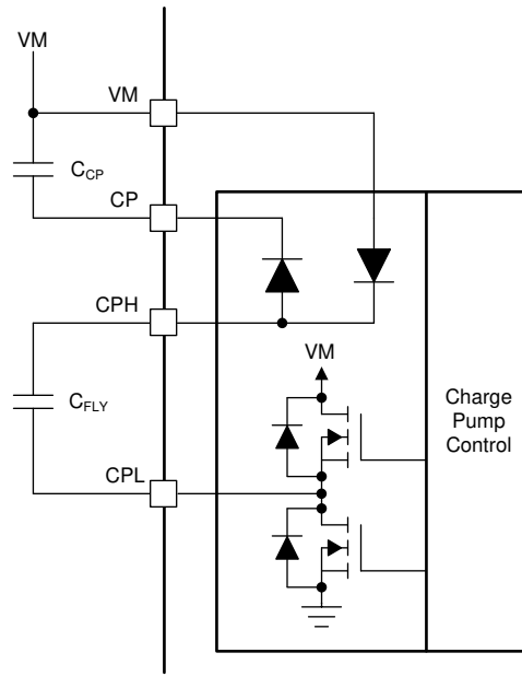
图 8-9. Charge Pump
