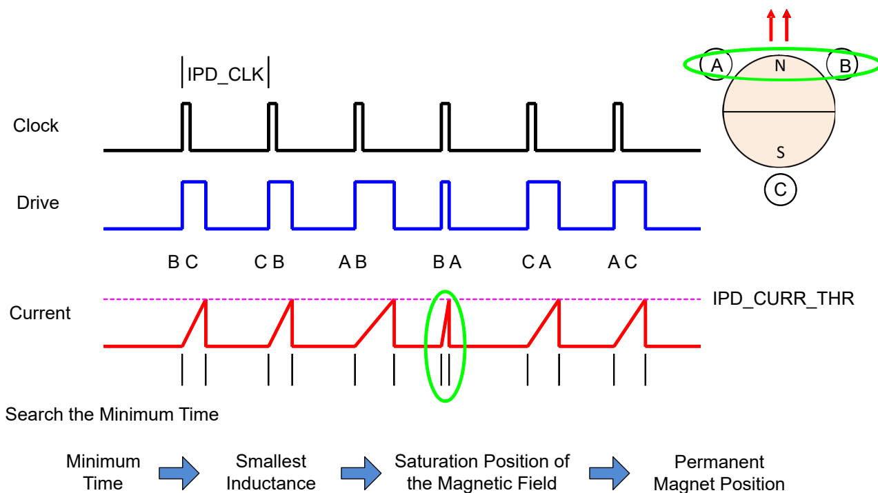
图 8-21. IPD Function
